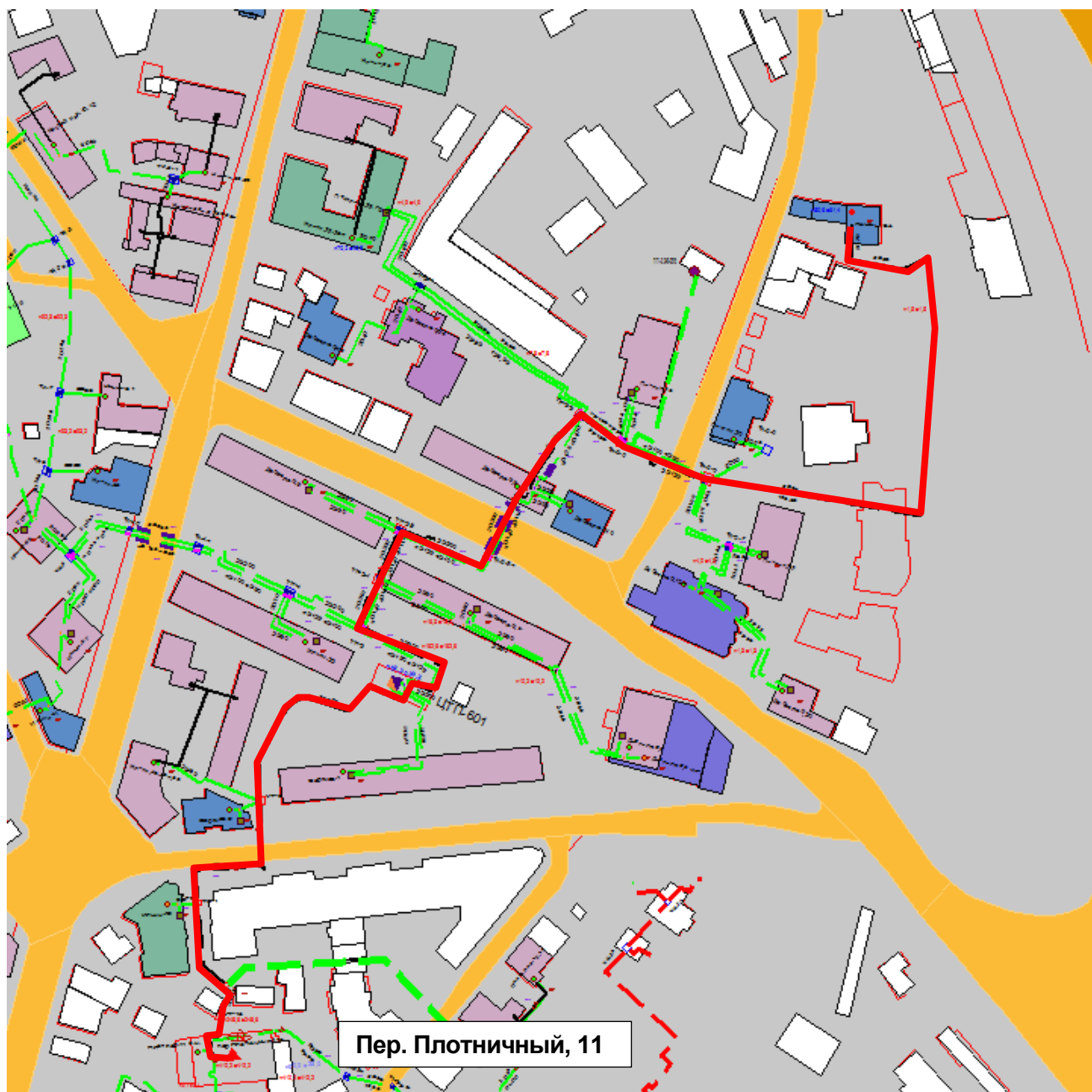
Рисунок Ошибка! Текст указанного стиля в документе отсутствует.185 – Результат гидравлического расчета - расчетный путь теплоносителя от котельной пер. Плотничный, 11 до ПТ-Почаин, 14а
