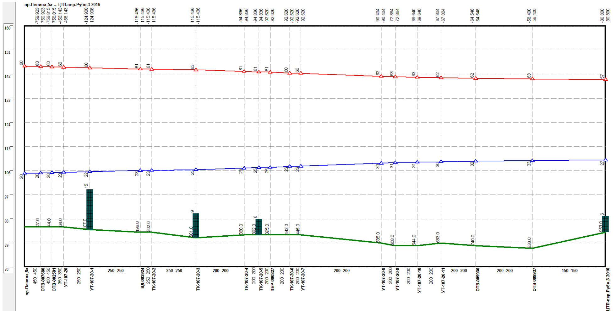
Рисунок Ошибка! Текст указанного стиля в документе отсутствует..190 –Результат гидравлического расчета - график гидравлических режимов по пути теплоносителя от котельной пр.Ленина, 5-а до ЦТП-пер.Рубо,3 2016
