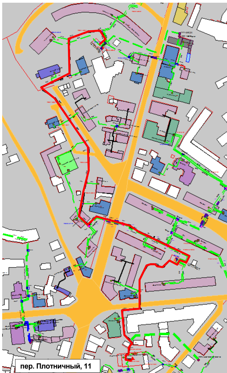
Рисунок Ошибка! Текст указанного стиля в документе отсутствует..183 – Результат гидравлического расчета - расчетный путь теплоносителя от котельной пер. Плотничный, 11 до ЦТП-602
