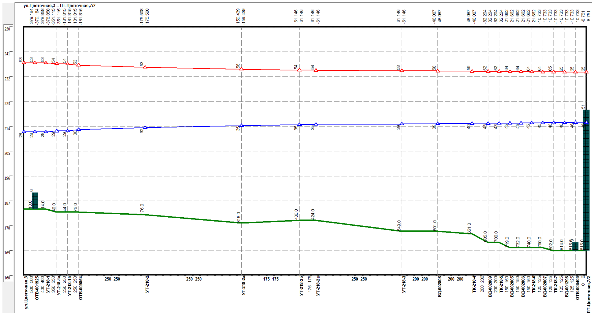
Рисунок Ошибка! Текст указанного стиля в документе отсутствует..222 –Результат гидравлического расчета - график гидравлических режимов по пути теплоносителя от котельной Цветочная, 3-а до ПТ-Цветочная, 7/2
