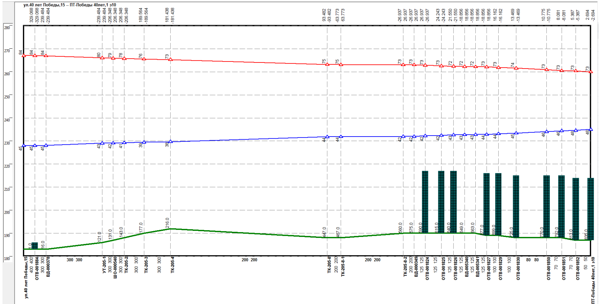
Рисунок Ошибка! Текст указанного стиля в документе отсутствует..202 –Результат гидравлического расчета - график гидравлических режимов по пути теплоносителя от котельной 40 лет Победы, д.15 до ПТ-Победа 40лет,1 э10
