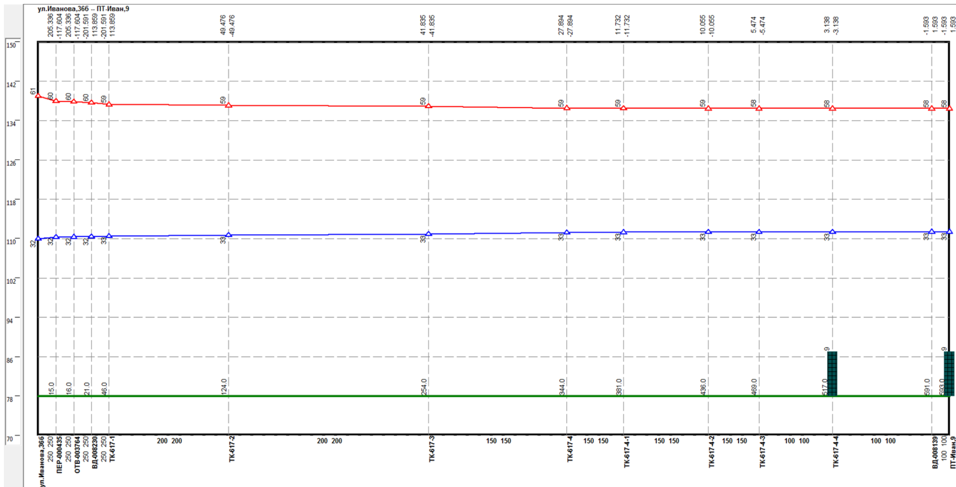
Рисунок Ошибка! Текст указанного стиля в документе отсутствует..210 –Результат гидравлического расчета - график гидравлических режимов по пути теплоносителя от котельной Иванова, 36-б до ПТ-Иван,9
