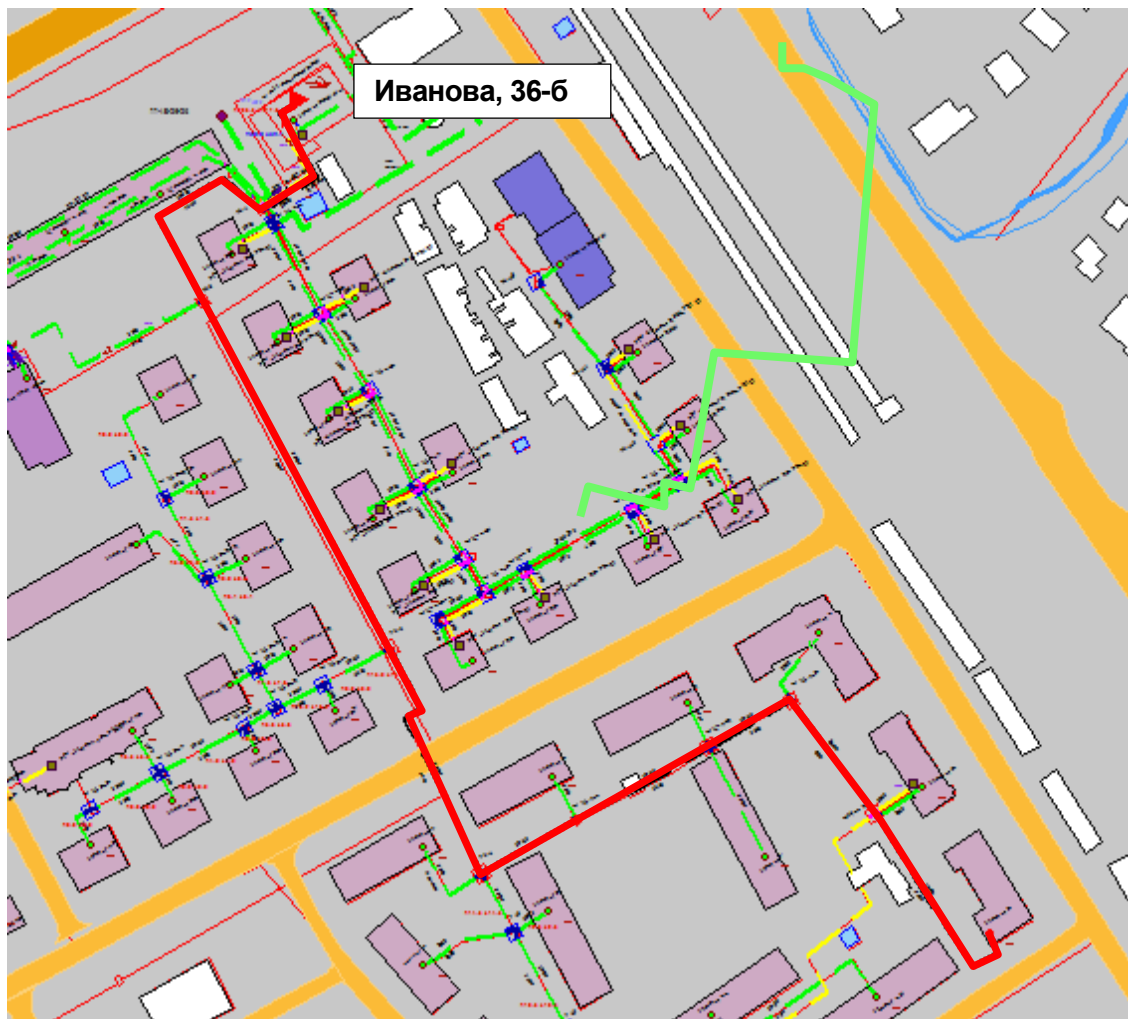
Рисунок Ошибка! Текст указанного стиля в документе отсутствует..209 – Результат гидравлического расчета - расчетный путь теплоносителя от котельной Иванова, 36-б до ПТ-Иван,9
