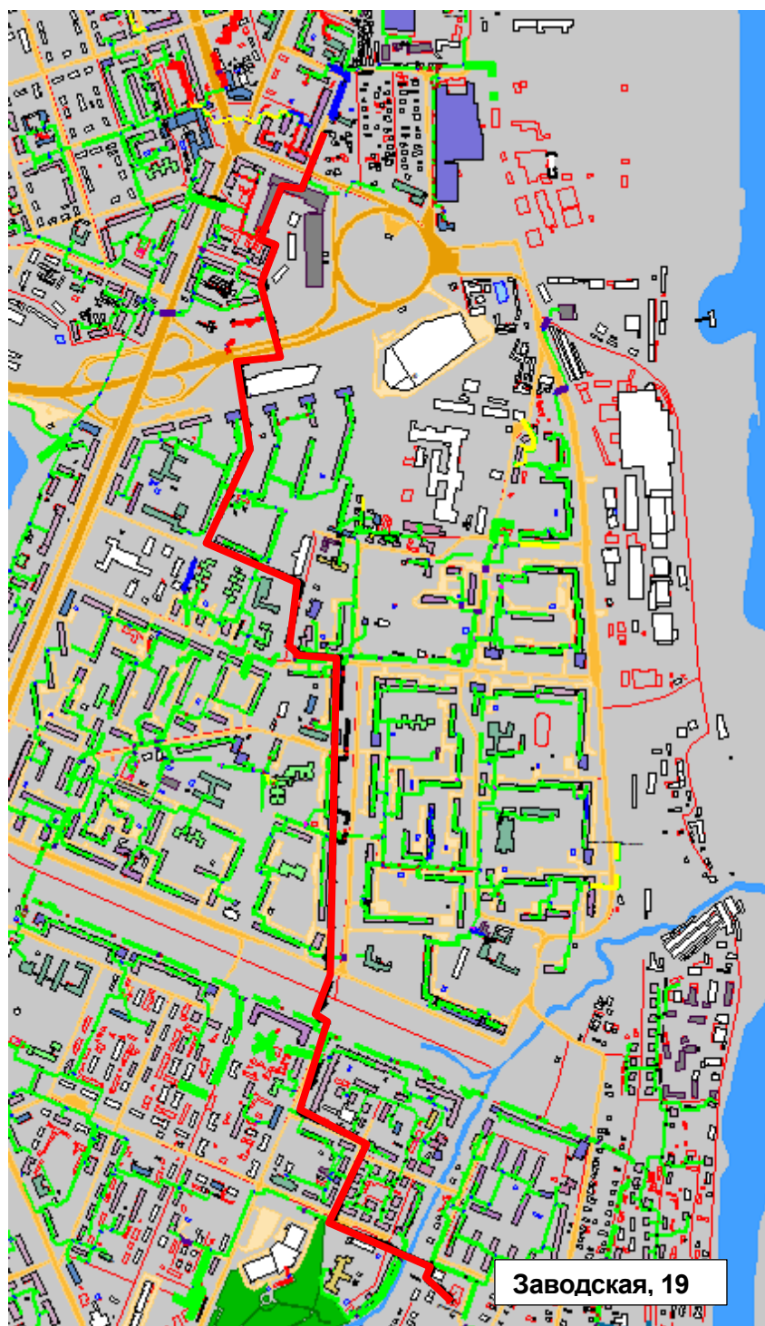
Рисунок Ошибка! Текст указанного стиля в документе отсутствует..165 – Результат гидравлического расчета - расчетный путь теплоносителя от котельной ФГУП НПП «Полет» до ПТ-Мичур,2
