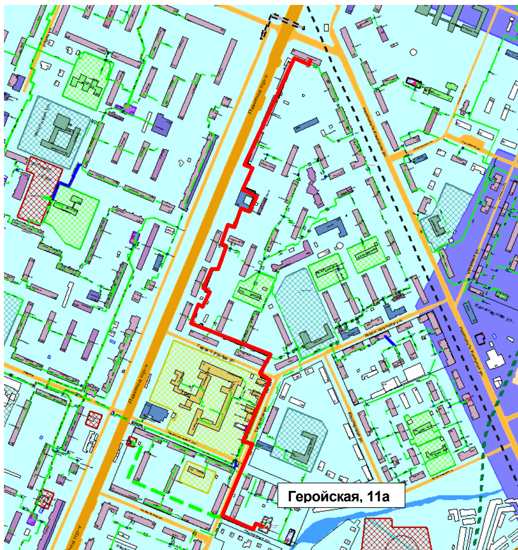
Рисунок Ошибка! Текст указанного стиля в документе отсутствует..161 – Результат гидравлического расчета - расчетный путь теплоносителя от котельной Геройская, 11а до ПТ-пр. Ленина, 38
