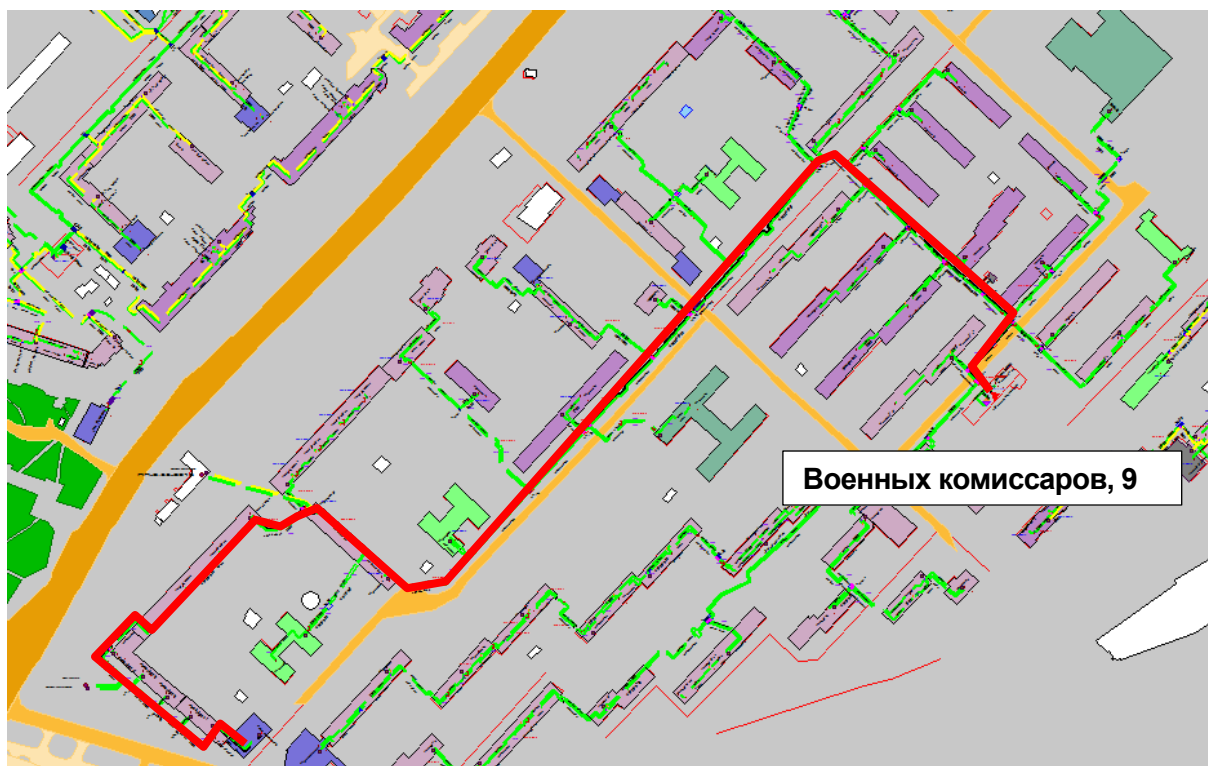
Рисунок Ошибка! Текст указанного стиля в документе отсутствует..203 – Результат гидравлического расчета - расчетный путь теплоносителя от от котельной Военных комиссаров, 9 до ПТ-Гагар.пр,226 пристр
