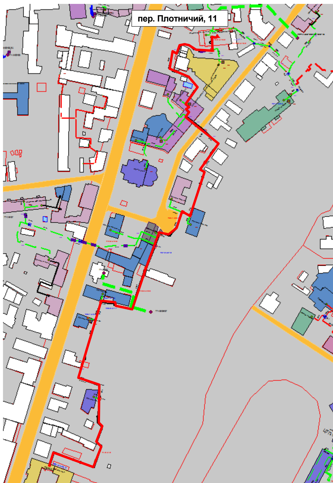
Рисунок Ошибка! Текст указанного стиля в документе отсутствует..181 – Результат гидравлического расчета - расчетный путь теплоносителя от котельной пер. Плотничий, 11 до ПТ-Ильин,78,78а,гар
