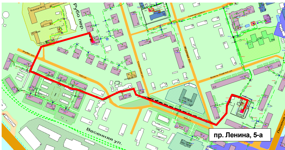
Рисунок Ошибка! Текст указанного стиля в документе отсутствует.189 – Результат гидравлического расчета - расчетный путь теплоносителя от котельной пр. Ленина, 5-а до ЦТП-пер.Рубо,3 2016
