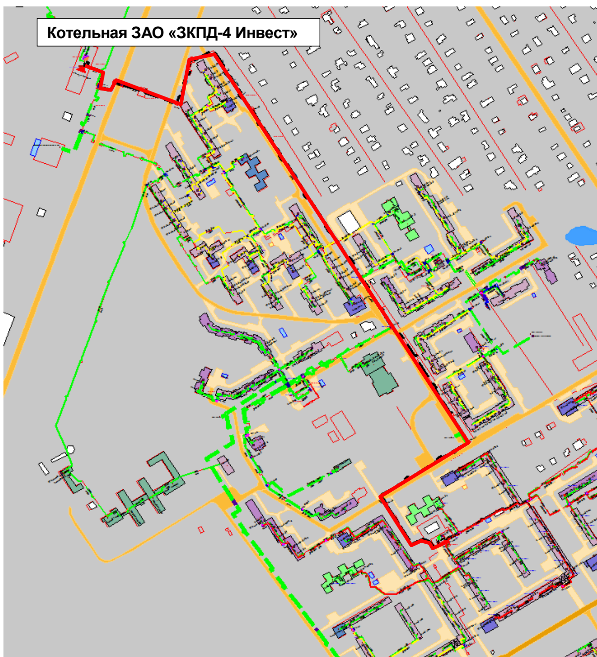
Рисунок 1.149- Результат гидравлического расчета - расчетный путь теплоносителя от котельной ЗАО «ЗКПД-4 Инвест» до ПТ-Кораб,26/2 аптека Основные характеристики теплопровода и режимные параметры теплоносителя приведены в таблице 1.117.
