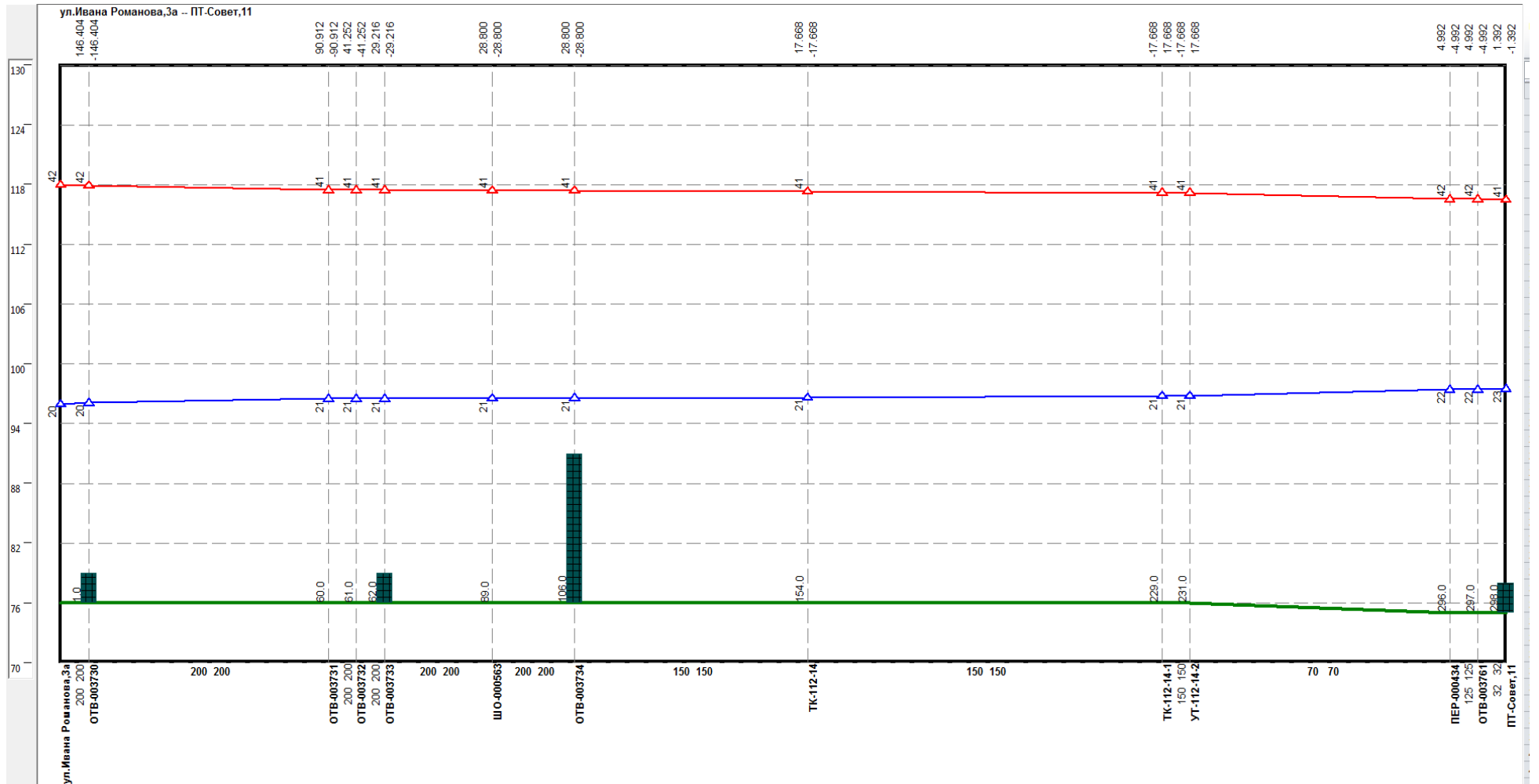
Рисунок Ошибка! Текст указанного стиля в документе отсутствует..144 –Результат гидравлического расчета - график гидравлических режимов по пути теплоносителя от котельной Ивана Романова до ПТ-Совет,11
