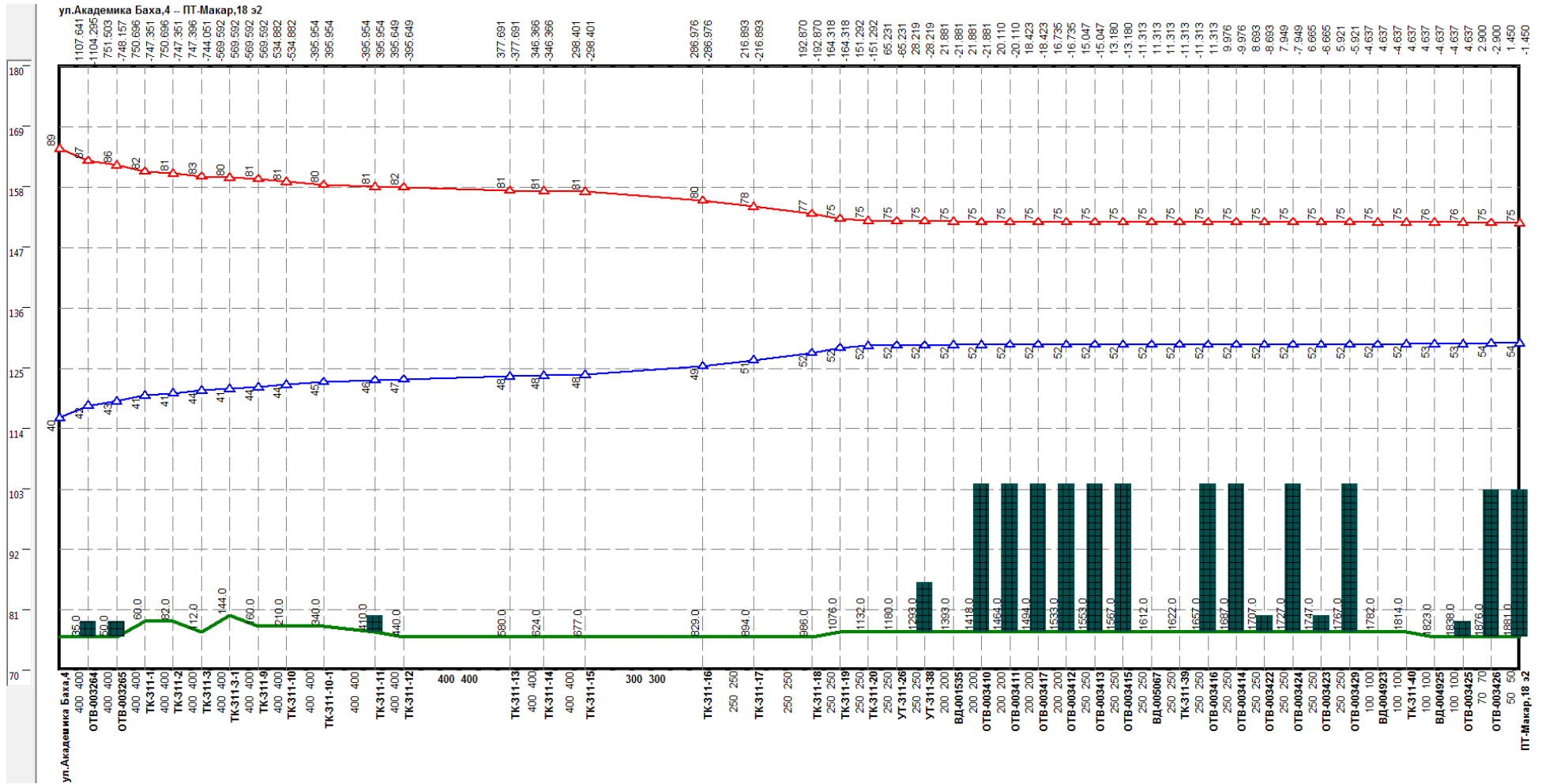
Рисунок Ошибка! Текст указанного стиля в документе отсутствует..208 –Результат гидравлического расчета - график гидравлических режимов по пути теплоносителя от котельной Академика Баха, 4-а до ПТ-Макар,18 э2
