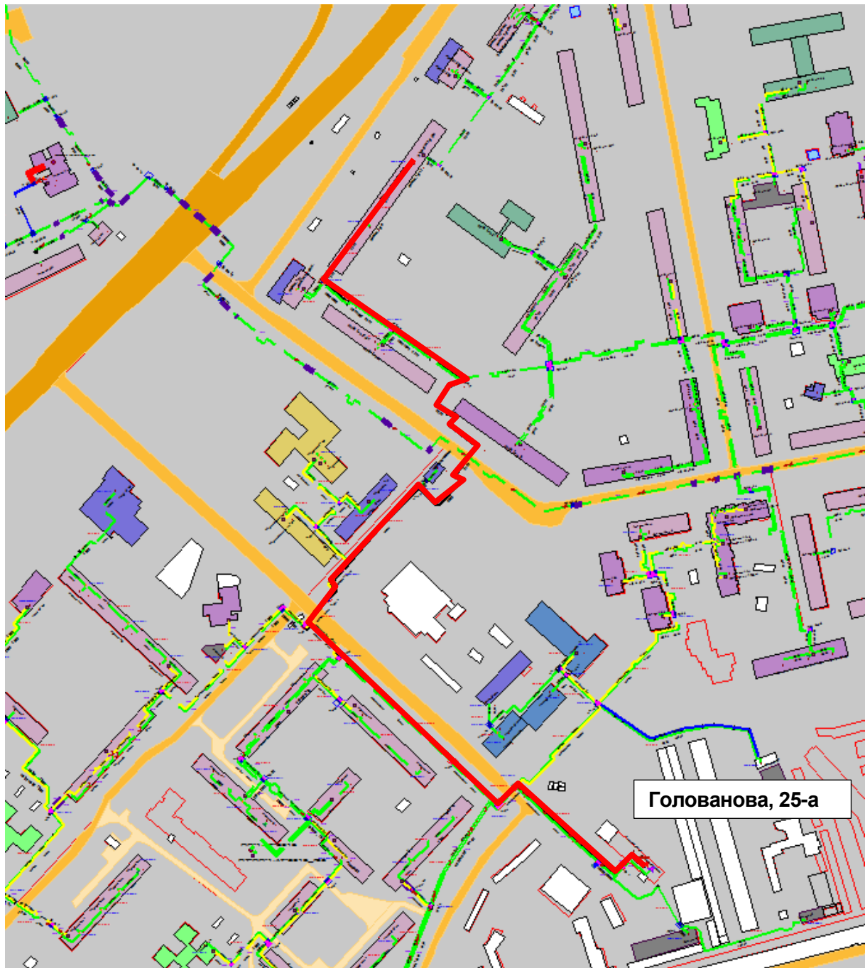
Рисунок Ошибка! Текст указанного стиля в документе отсутствует..213 – Результат гидравлического расчета - расчетный путь теплоносителя от котельной Голованова, 25-а до ПТ-Гагар.пр,184 э2
