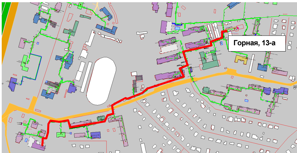
Рисунок Ошибка! Текст указанного стиля в документе отсутствует..177 – Результат гидравлического расчета - расчетный путь теплоносителя от котельной Горная, 13-а до ПТ-Горная,2(стр.)
