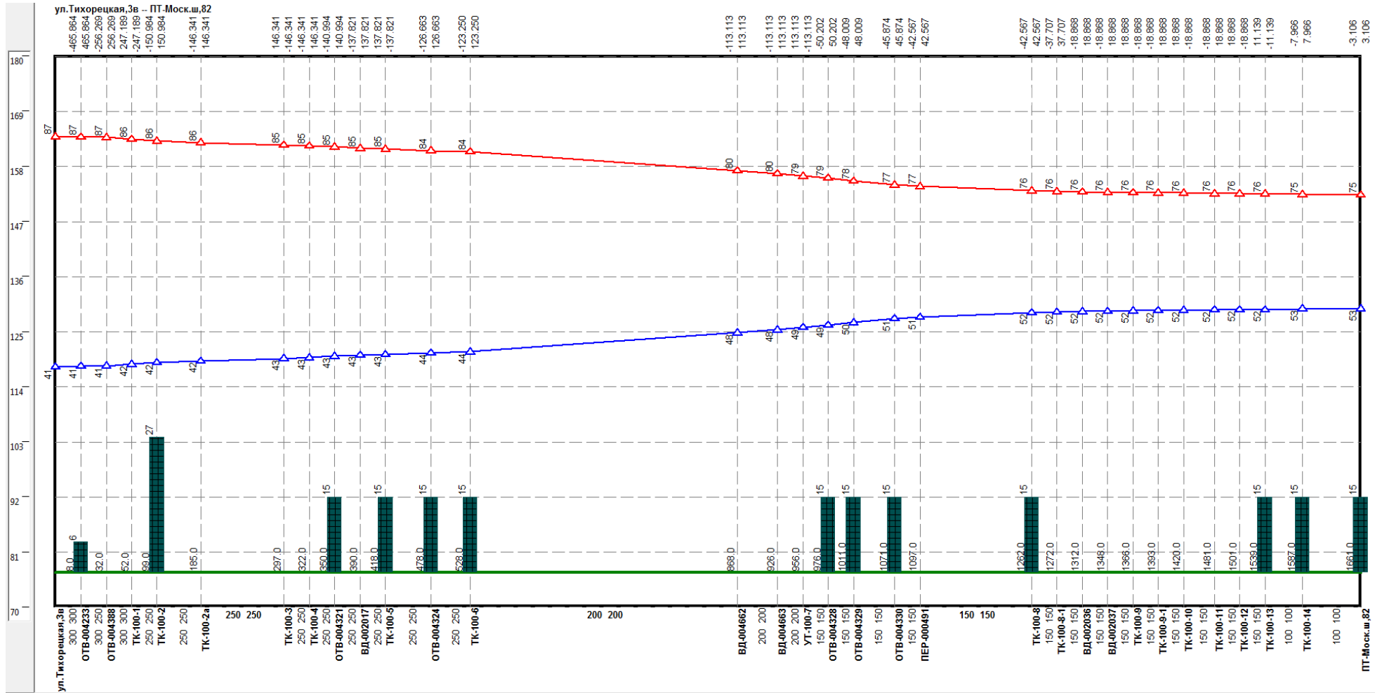
Рисунок Ошибка! Текст указанного стиля в документе отсутствует..168 –Результат гидравлического расчета - график гидравлических режимов по пути теплоносителя от котельной Тихорецкая, 3-в до ПТ-Моск.ш.82
