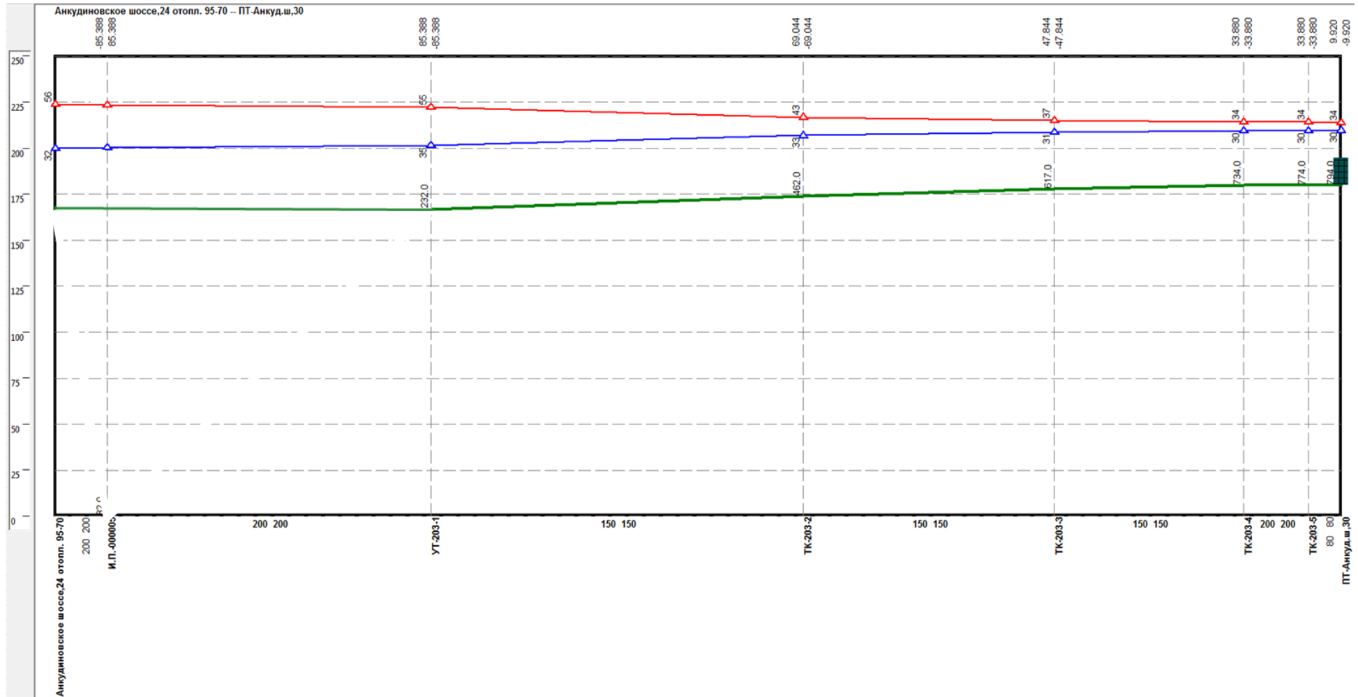
Рисунок Ошибка! Текст указанного стиля в документе отсутствует..192 –Результат гидравлического расчета - график гидравлических режимов по пути теплоносителя от котельной Анкудиновское шоссе, 24 до ПТ-Анкуд.ш,30
