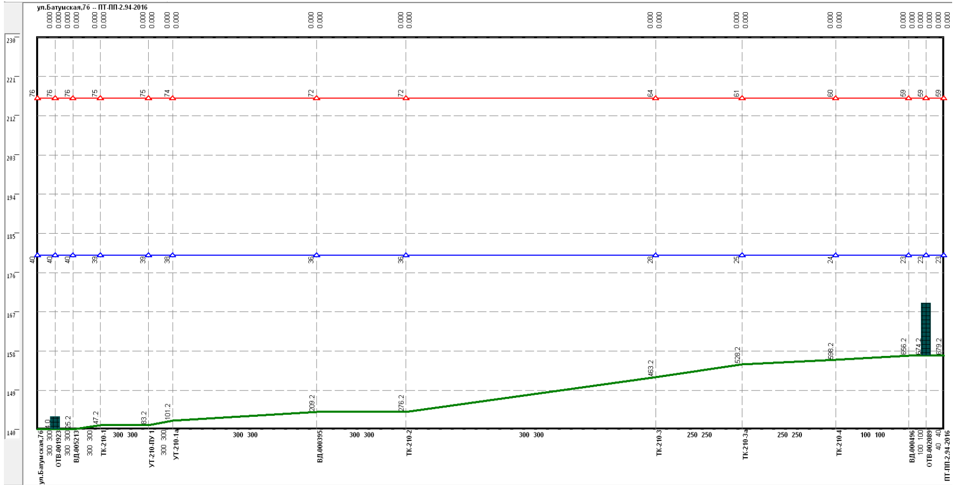
Рисунок Ошибка! Текст указанного стиля в документе отсутствует..158 –Результат гидравлического расчета - график гидравлических режимов по пути теплоносителя от котельной Батумская, 76 до ПТ-ПП-2.94-2016
