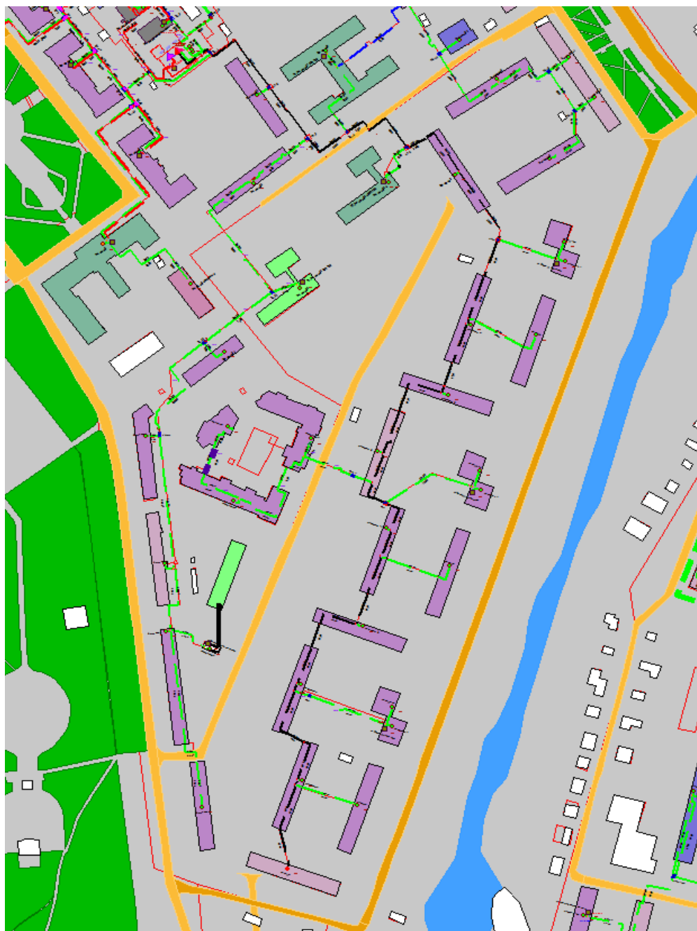
Рисунок Ошибка! Текст указанного стиля в документе отсутствует..199 – Результат гидравлического расчета - расчетный путь теплоносителя от котельной Энгельса, 1-в до ПТ-Больш,7
