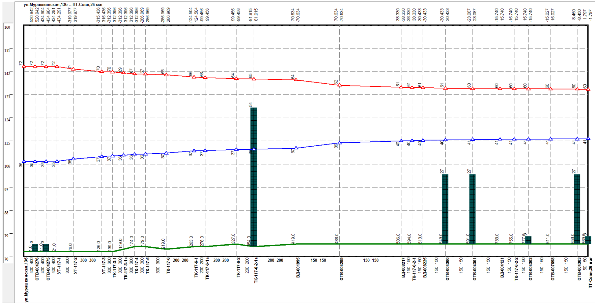
Рисунок Ошибка! Текст указанного стиля в документе отсутствует..152 –Результат гидравлического расчета - график гидравлических режимов по пути теплоносителя от котельной Мурашкинская, 13-б до ПТ-Совн,26 маг
