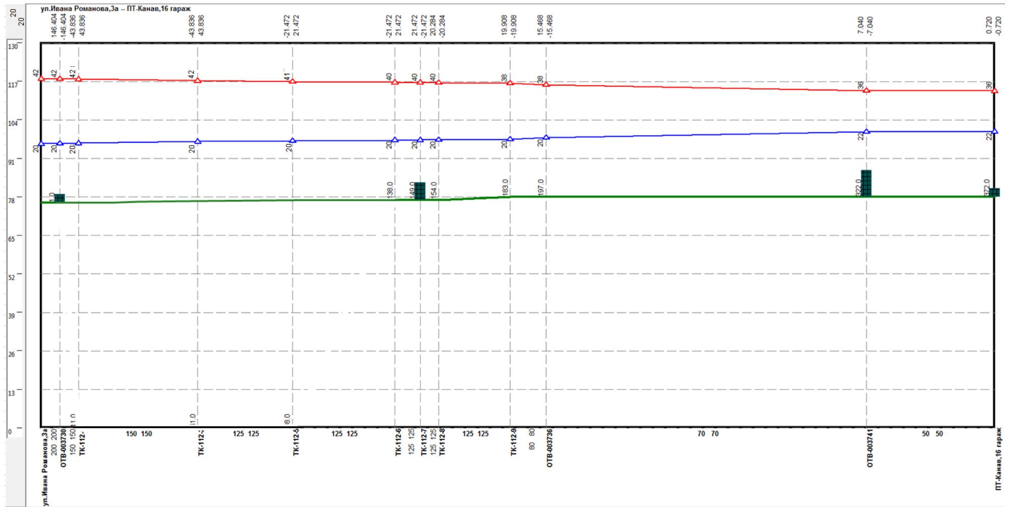
Рисунок Ошибка! Текст указанного стиля в документе отсутствует..146 –Результат гидравлического расчета - график гидравлических режимов по пути теплоносителя от котельной Ивана Романова, За до ПТ-Канав,16 гараж
