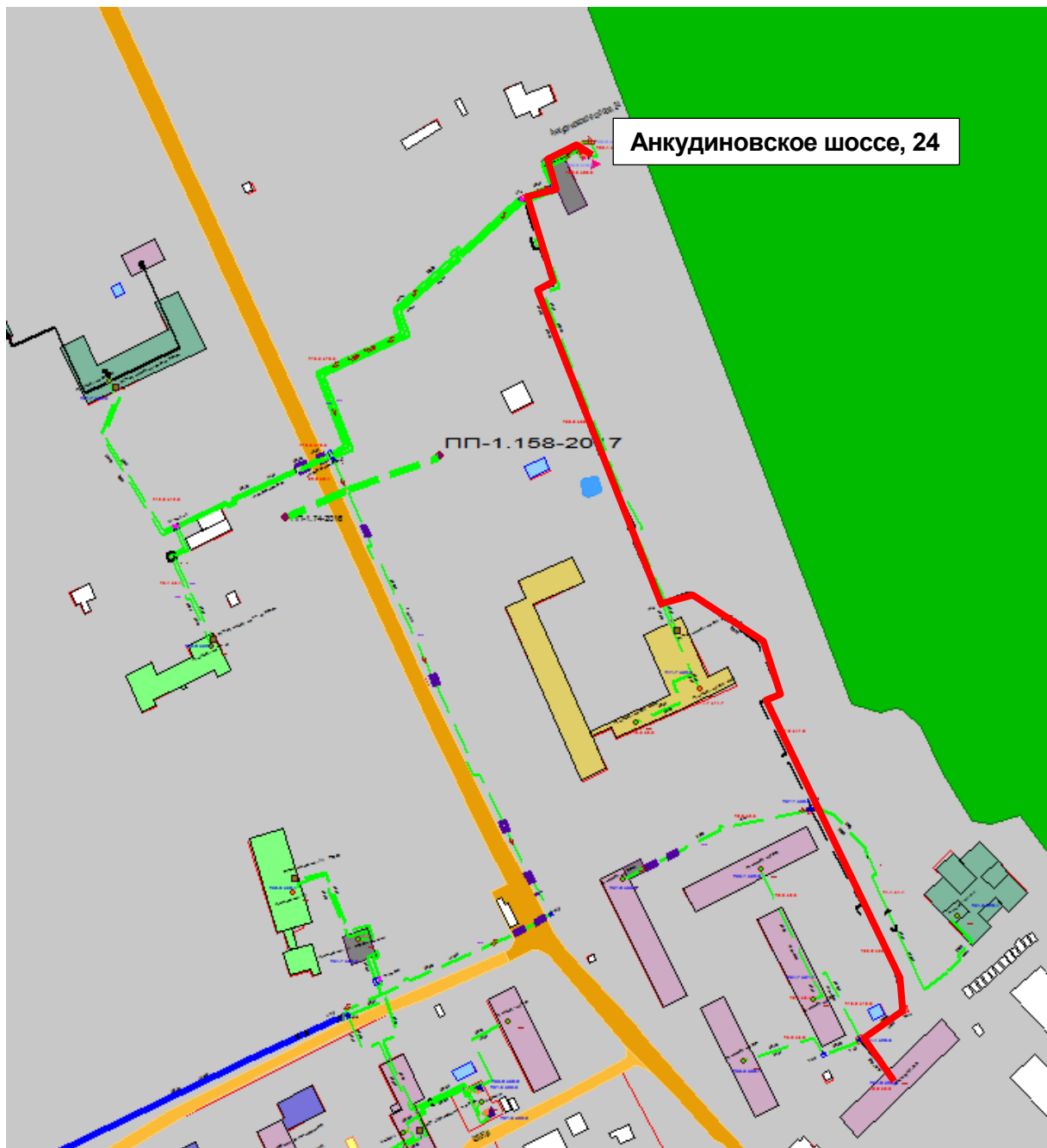
Рисунок Ошибка! Текст указанного стиля в документе отсутствует..191 – Результат гидравлического расчета - расчетный путь теплоносителя от котельной Анкудиновское шоссе, 24 до ПТ-Анкуд.ш,30
