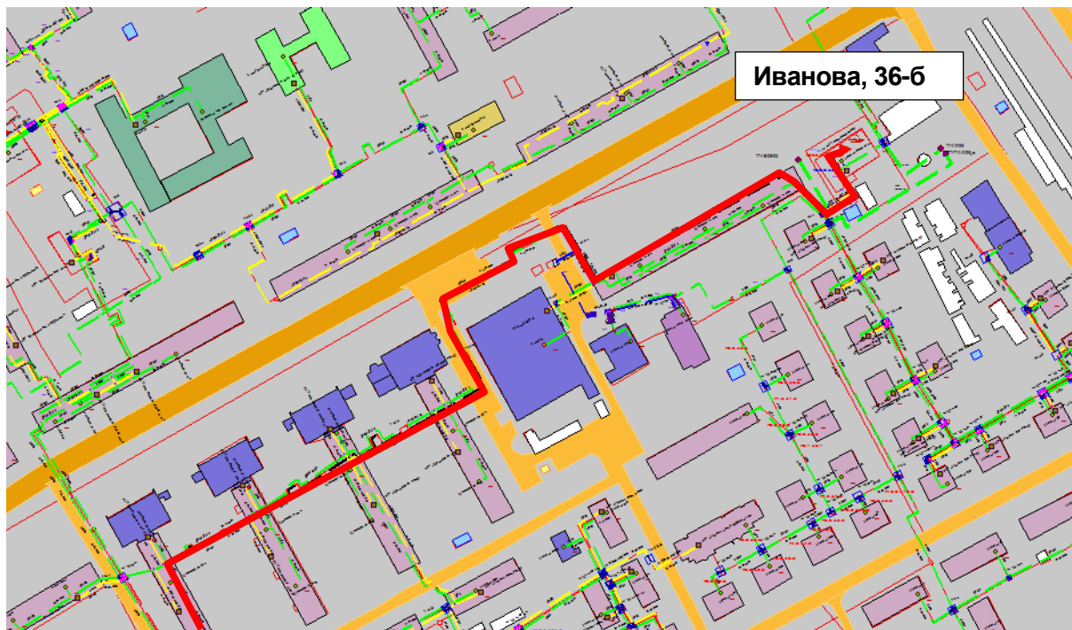
Рисунок Ошибка! Текст указанного стиля в документе отсутствует..211 – Результат гидравлического расчета - расчетный путь теплоносителя от котельной Иванова, 36-б до ПТ-Кораб,9 Э2
