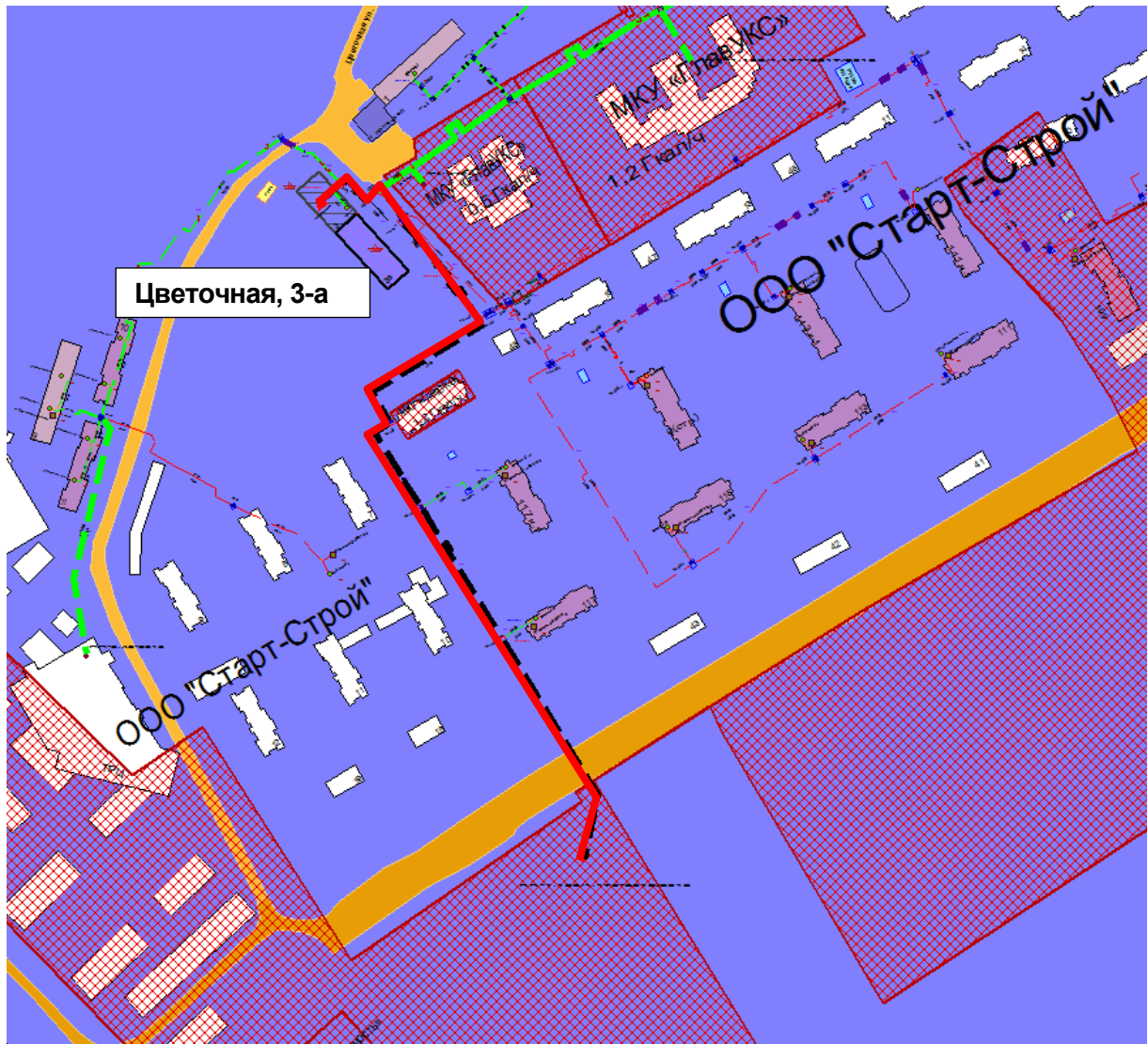
Рисунок Ошибка! Текст указанного стиля в документе отсутствует..223 – Результат гидравлического расчета - расчетный путь теплоносителя от котельной Цветочная, 3-а до ПТ-Гаугеля,1 до ПТ-ПП-1.150/1.170-2016/2018
