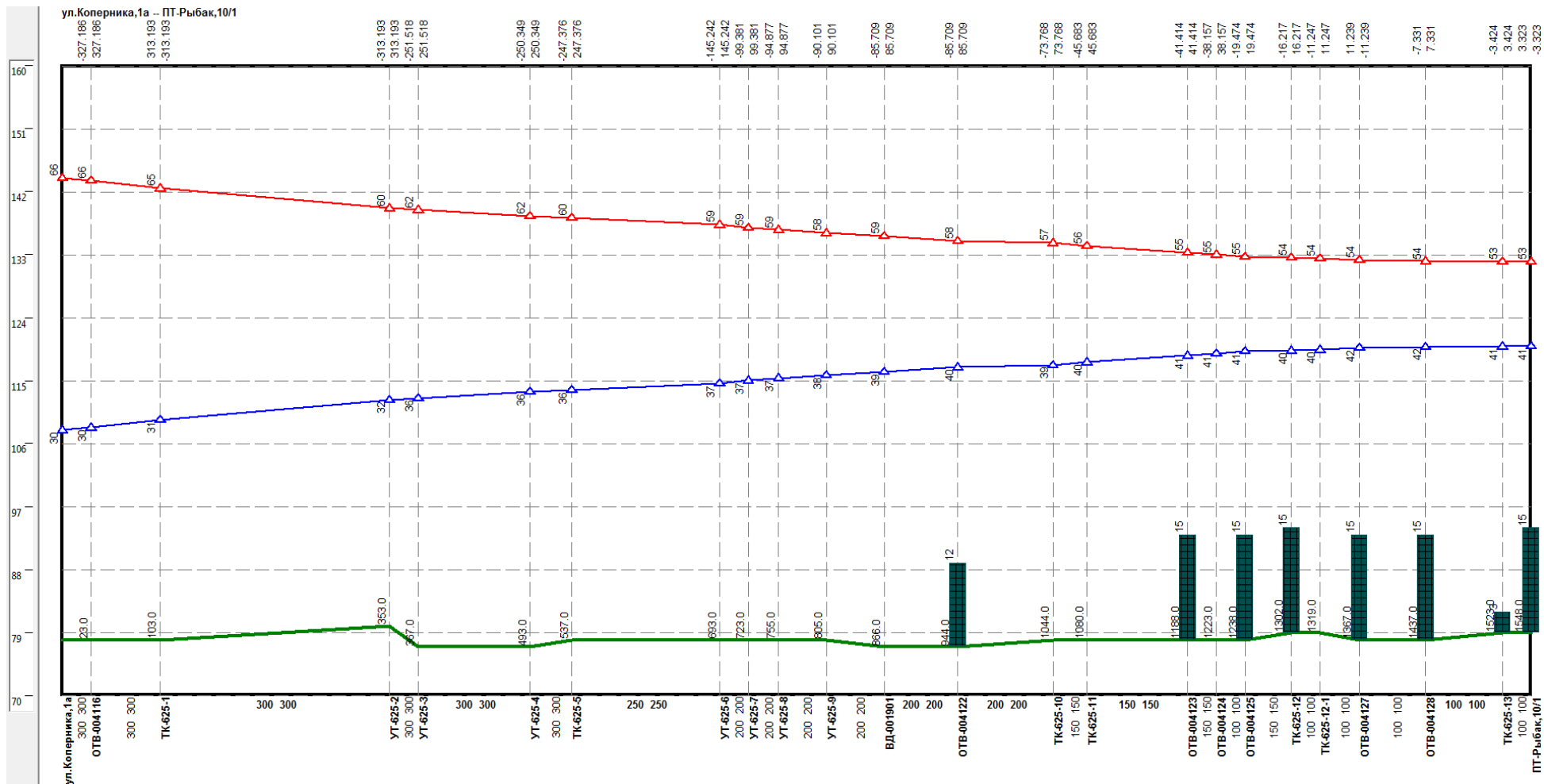
Рисунок Ошибка! Текст указанного стиля в документе отсутствует..220 –Результат гидравлического расчета - график гидравлических режимов по пути теплоносителя от котельной Коперника, 1-а до ПТ-Рыбак,10/1
