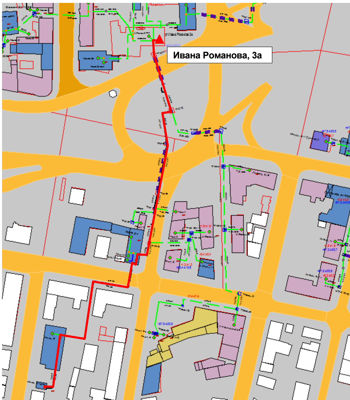
Рисунок Ошибка! Текст указанного стиля в документе отсутствует..145 - Результат гидравлического расчета - расчетный путь теплоносителя от котельной Ивана Романова, 3а до ПТ-Канав,16 гараж
