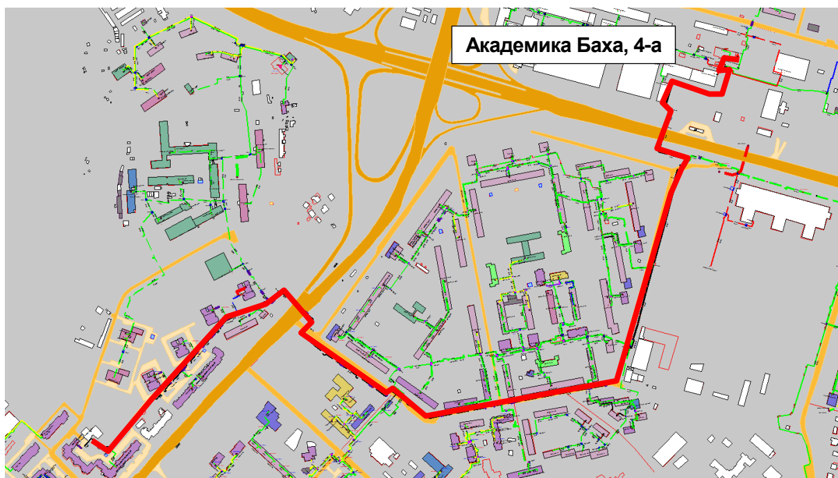
Рисунок Ошибка! Текст указанного стиля в документе отсутствует..207 – Результат гидравлического расчета - расчетный путь теплоносителя от котельной Академика Баха, 4-а до ПТ-Макар, 18 э2
