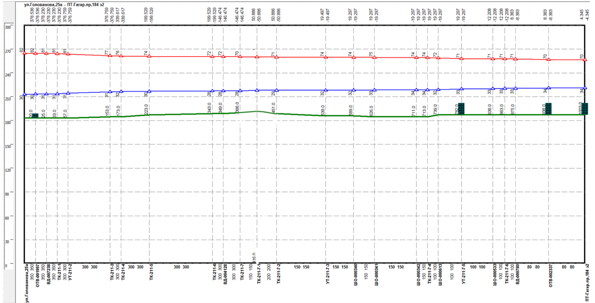
Рисунок Ошибка! Текст указанного стиля в документе отсутствует..214 –Результат гидравлического расчета - график гидравлических режимов по пути теплоносителя от котельной Голованова, 25-а до ПТ-Гагар.пр,184 э2
