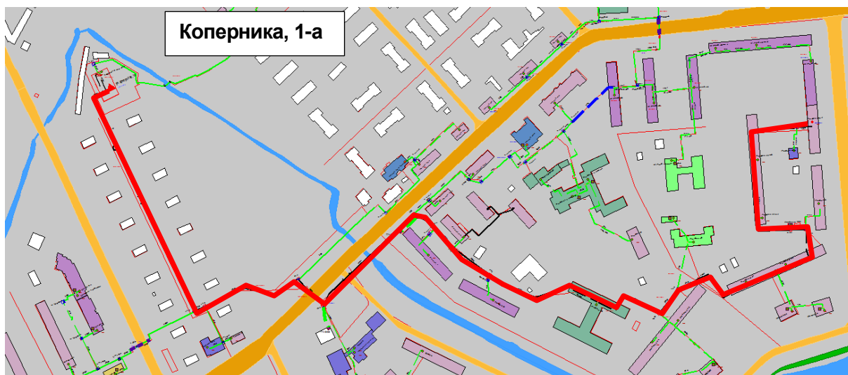
Рисунок Ошибка! Текст указанного стиля в документе отсутствует..219 – Результат гидравлического расчета - расчетный путь теплоносителя от котельной Коперника, 1-а до ПТ-Рыбак, 10/1
