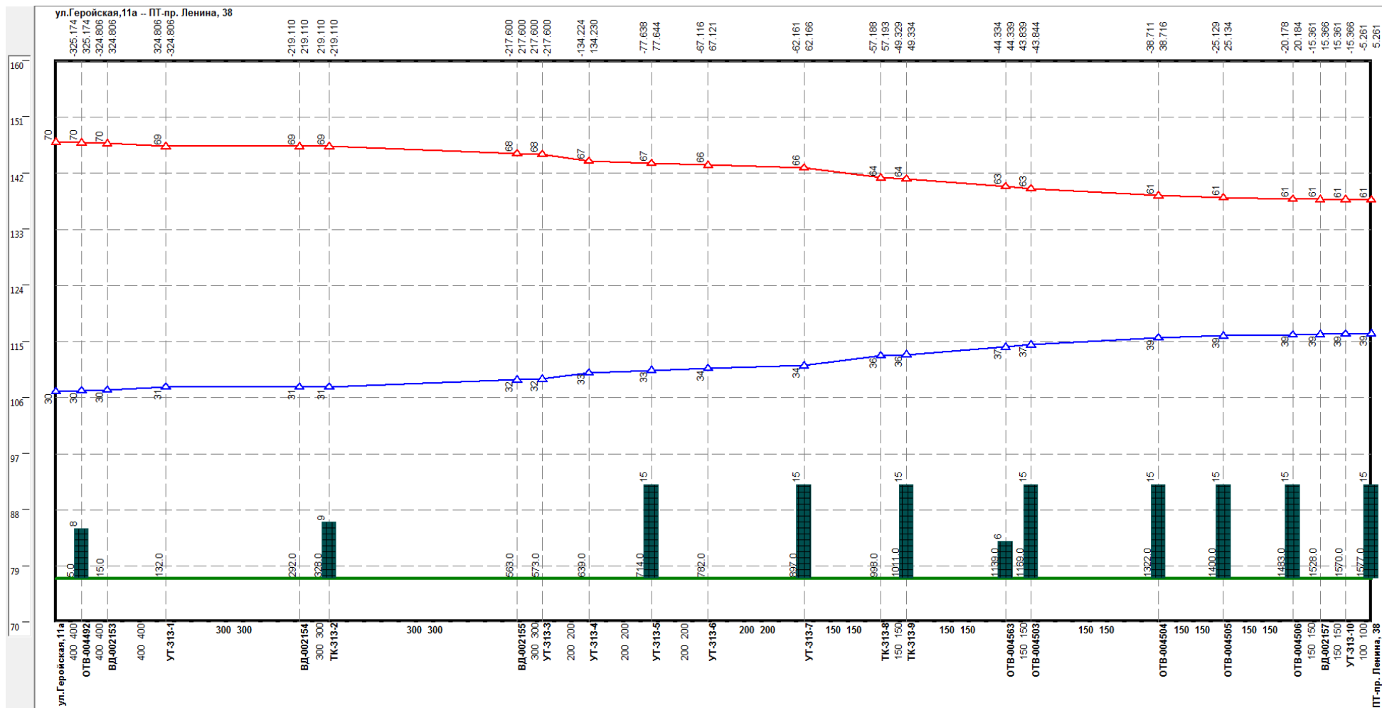
Рисунок Ошибка! Текст указанного стиля в документе отсутствует..162 –Результат гидравлического расчета - график гидравлических режимов по пути теплоносителя от котельной Геройская, 11а до ПТ-пр. Ленина, 38
