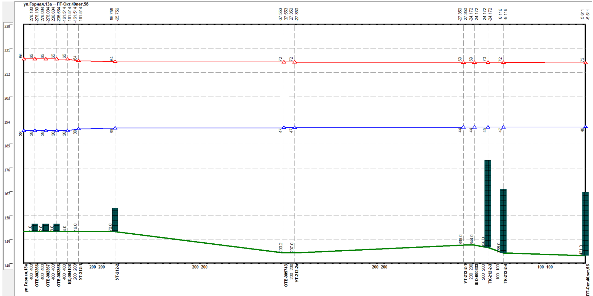
Рисунок Ошибка! Текст указанного стиля в документе отсутствует..180 –Результат гидравлического расчета - график гидравлических режимов по пути теплоносителя 2 от котельной Горная, 13-а до ПТ-Окт.40лет,56
