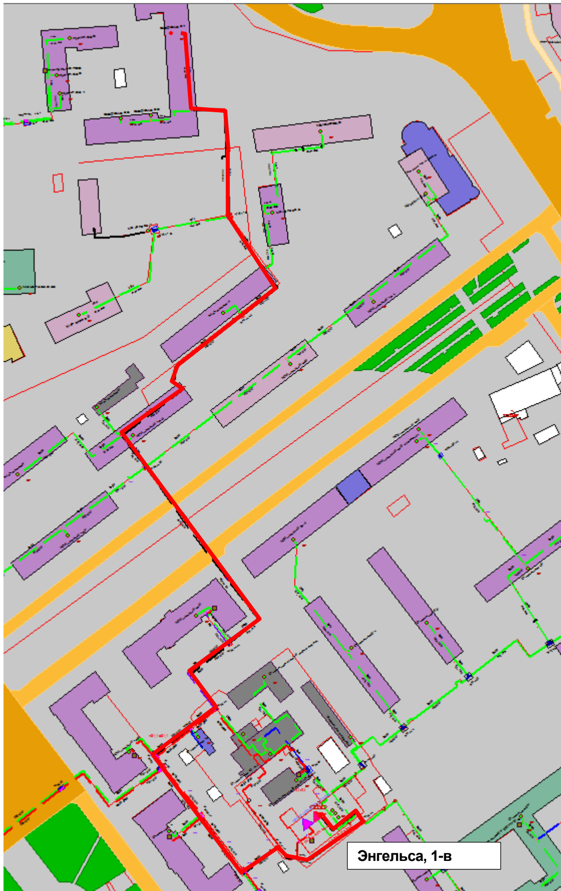
Рисунок Ошибка! Текст указанного стиля в документе отсутствует..195 – Результат гидравлического расчета - расчетный путь теплоносителя от котельной Энгельса, 1-в до ПТ-Ефрем,2 э1
