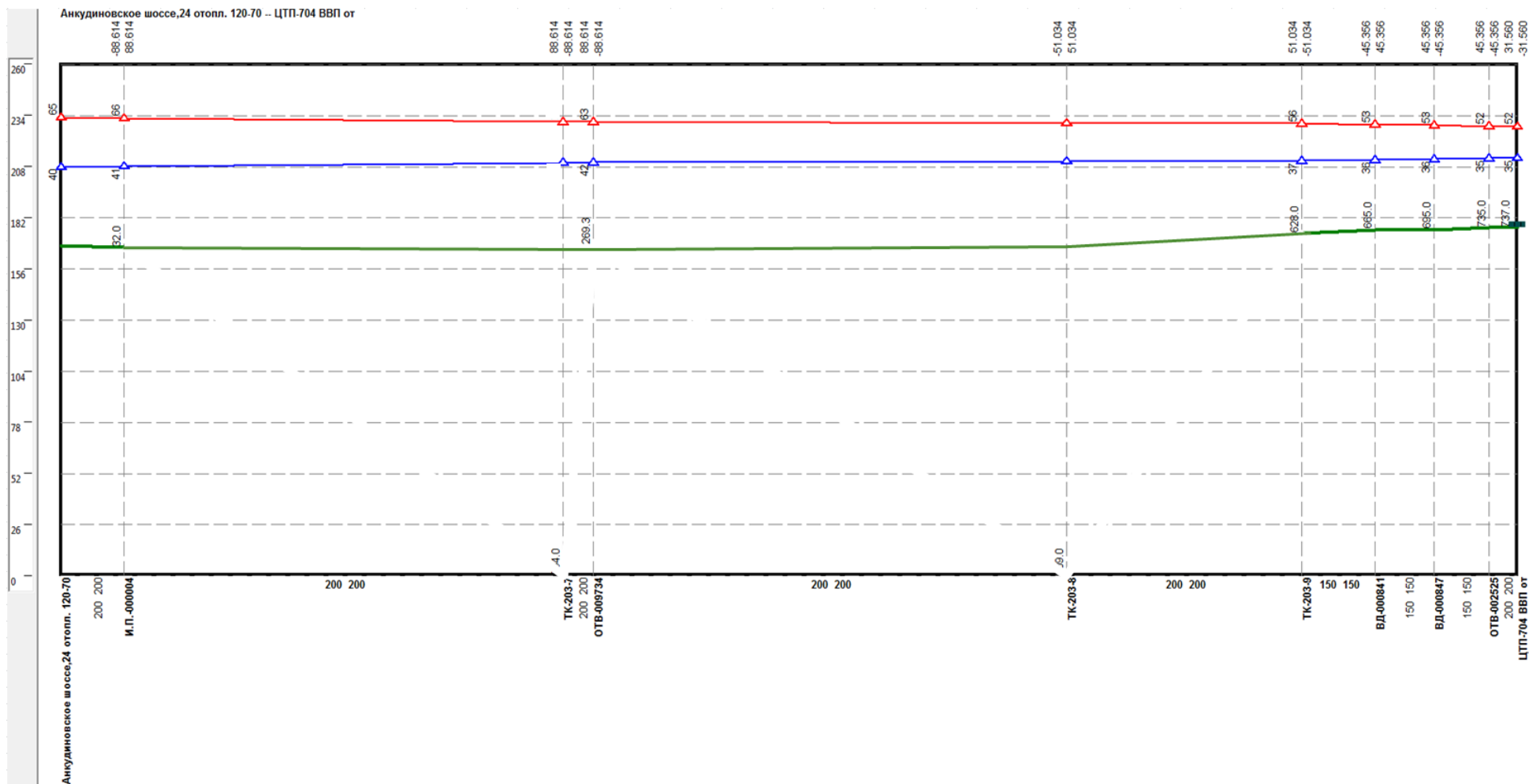
Рисунок Ошибка! Текст указанного стиля в документе отсутствует..194 –Результат гидравлического расчета - график гидравлических режимов по пути теплоносителя от котельной Анкудаиновское шоссе, 24 до ЦТП-704 ВВП от
