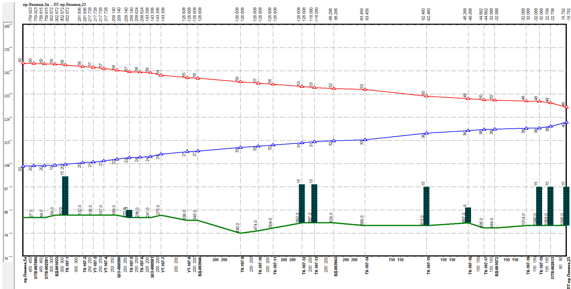
Рисунок Ошибка! Текст указанного стиля в документе отсутствует..188 –Результат гидравлического расчета - график гидравлических режимов по пути теплоносителя от котельной пр. Ленина, 5-а до ПТ-пр.Ленина,23
