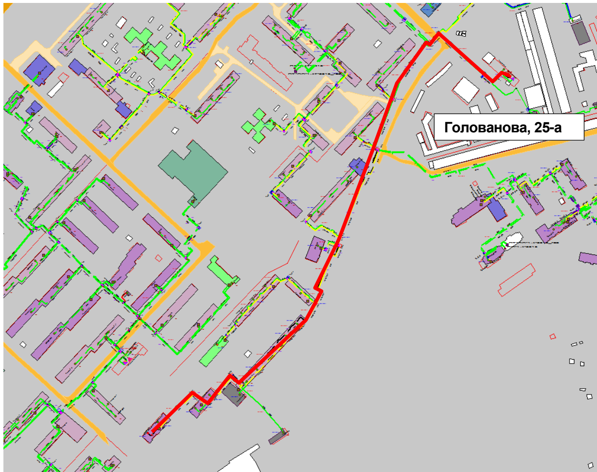
Рисунок Ошибка! Текст указанного стиля в документе отсутствует..215 – Результат гидравлического расчета - расчетный путь теплоносителя от котельной Голованова, 25-а до ПТ-Голован,57 э2
