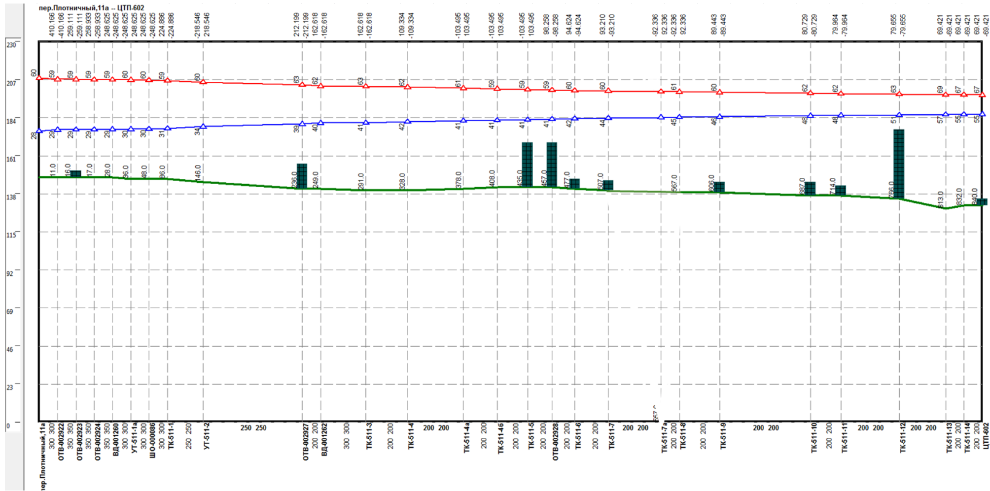
Рисунок Ошибка! Текст указанного стиля в документе отсутствует..184 –Результат гидравлического расчета - график гидравлических режимов по пути теплоносителя от котельной пер. Плотничный, 11 до ЦТП-602
