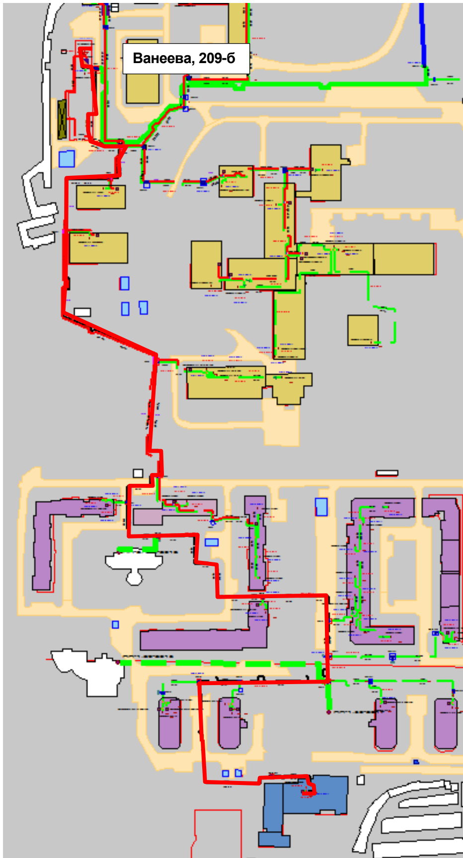
Рисунок Ошибка! Текст указанного стиля в документе отсутствует..175 – Результат гидравлического расчета - расчетный путь теплоносителя от котельной Ванеева, д.209-6 до ПТ-Ванеева_Пож.депо
