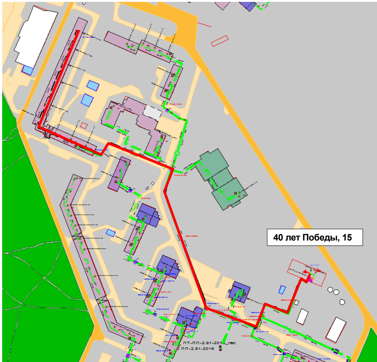
Рисунок Ошибка! Текст указанного стиля в документе отсутствует..201 – Результат гидравлического расчета - расчетный путь теплоносителя от котельной 40 лет Победы, д.15 до ПТ-Победы 40лет,1 з10
