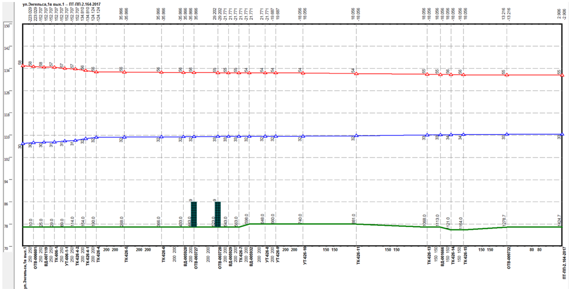
Рисунок Ошибка! Текст указанного стиля в документе отсутствует..198 – Результат гидравлического расчета - график гидравлических режимов по пути теплоносителя от котельной Энгельса, 1-в до ПТ-ПП-2.164.2017
