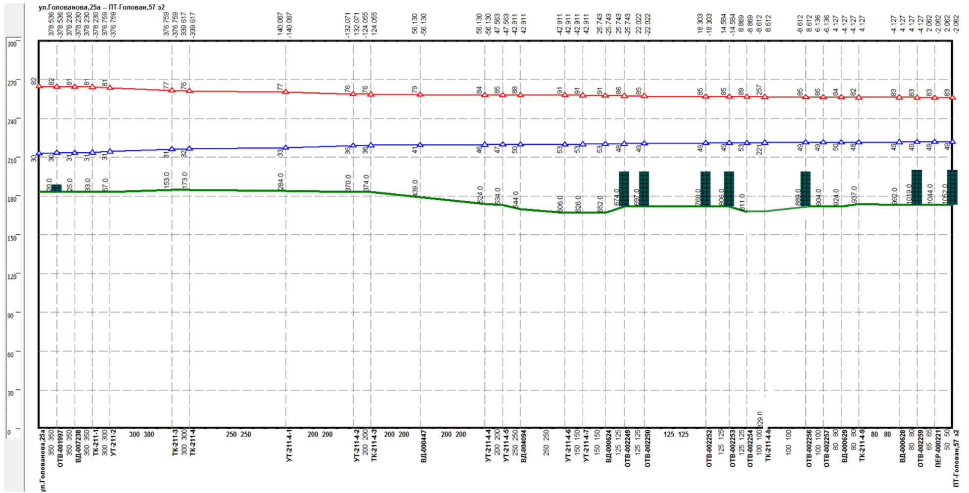
Рисунок Ошибка! Текст указанного стиля в документе отсутствует..216 –Результат гидравлического расчета - график гидравлических режимов по пути теплоносителя от котельной Голованова, 25-а до ПТ-Голован,57 э2
