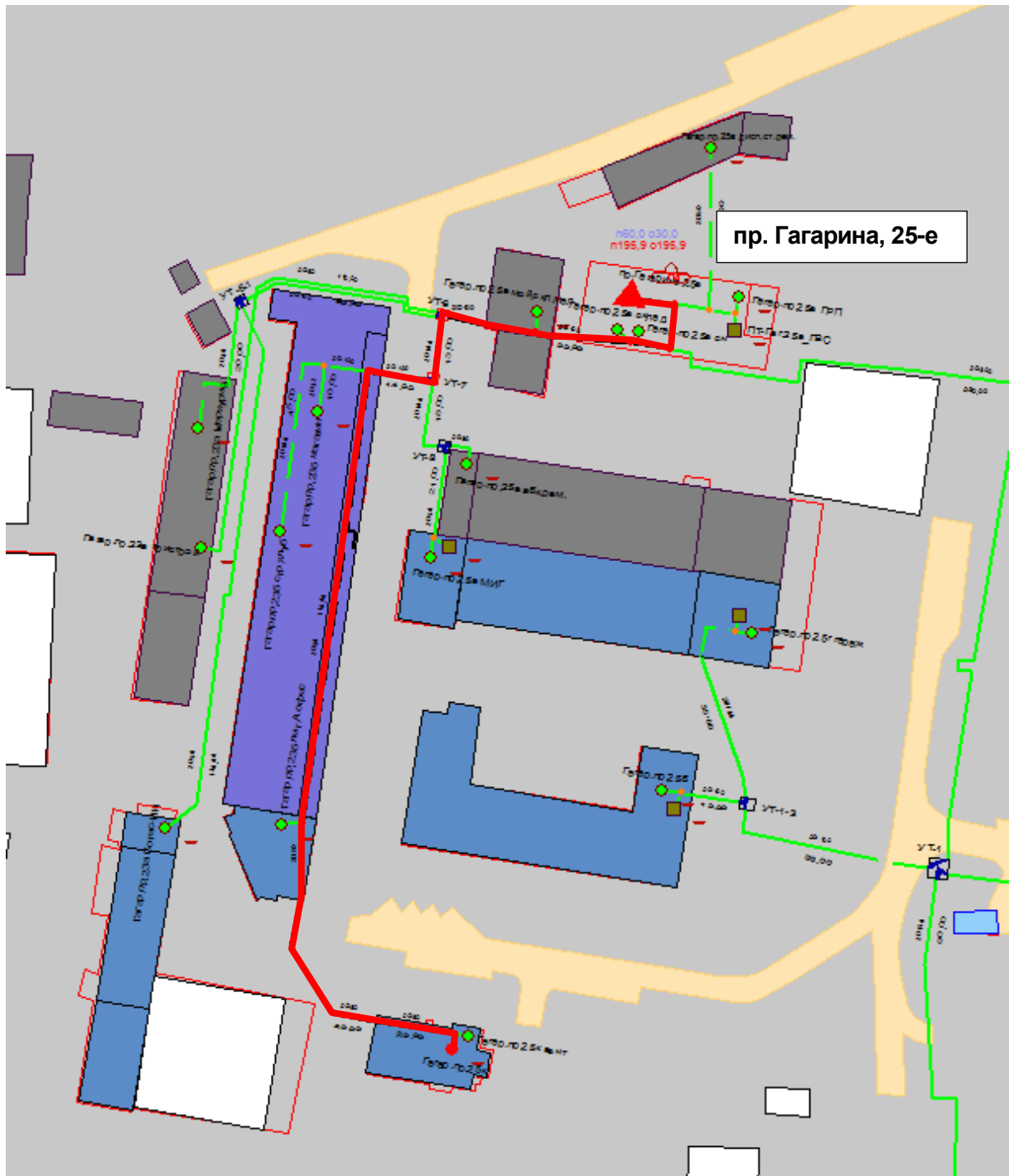
Рисунок Ошибка! Текст указанного стиля в документе отсутствует..173 – Результат гидравлического расчета - расчетный путь теплоносителя от котельной пр. Гагарина, 25-е до ПТ-Гагар.пр,31 хлор
