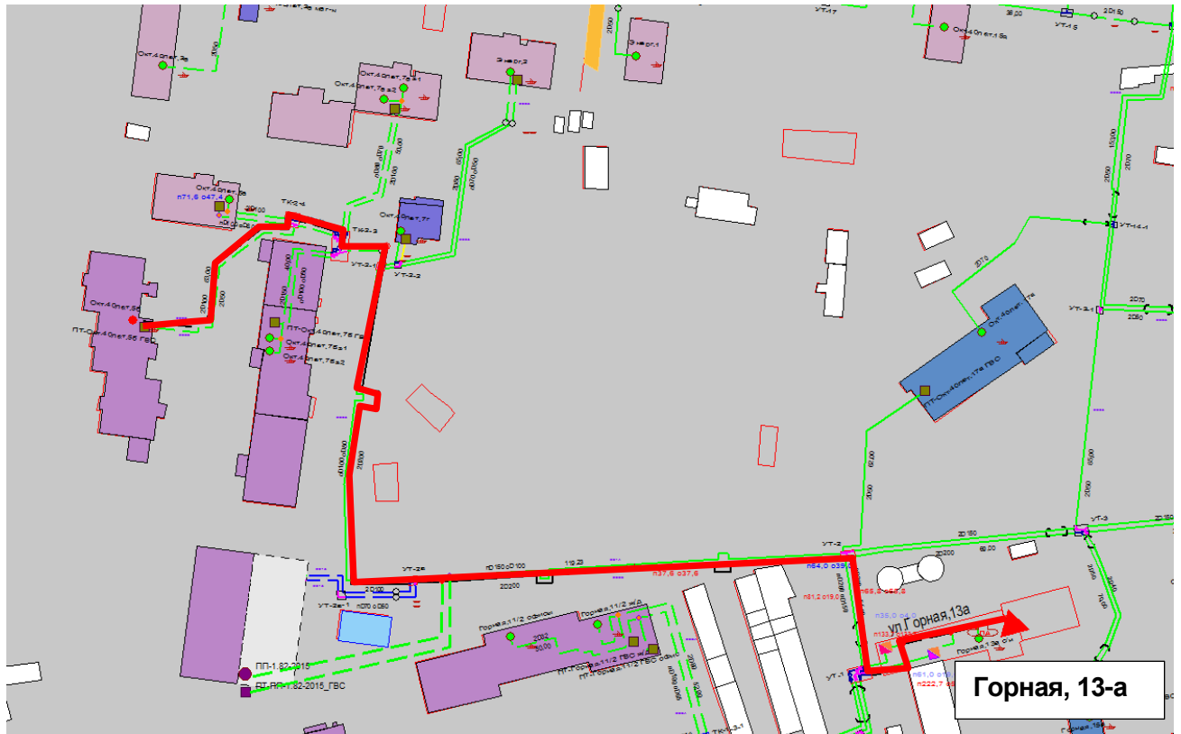
Рисунок Ошибка! Текст указанного стиля в документе отсутствует..179 – Результат гидравлического расчета - расчетный путь теплоносителя 2 от котельной Горная, 13-а до ПТ-Окт.40лет,5б
