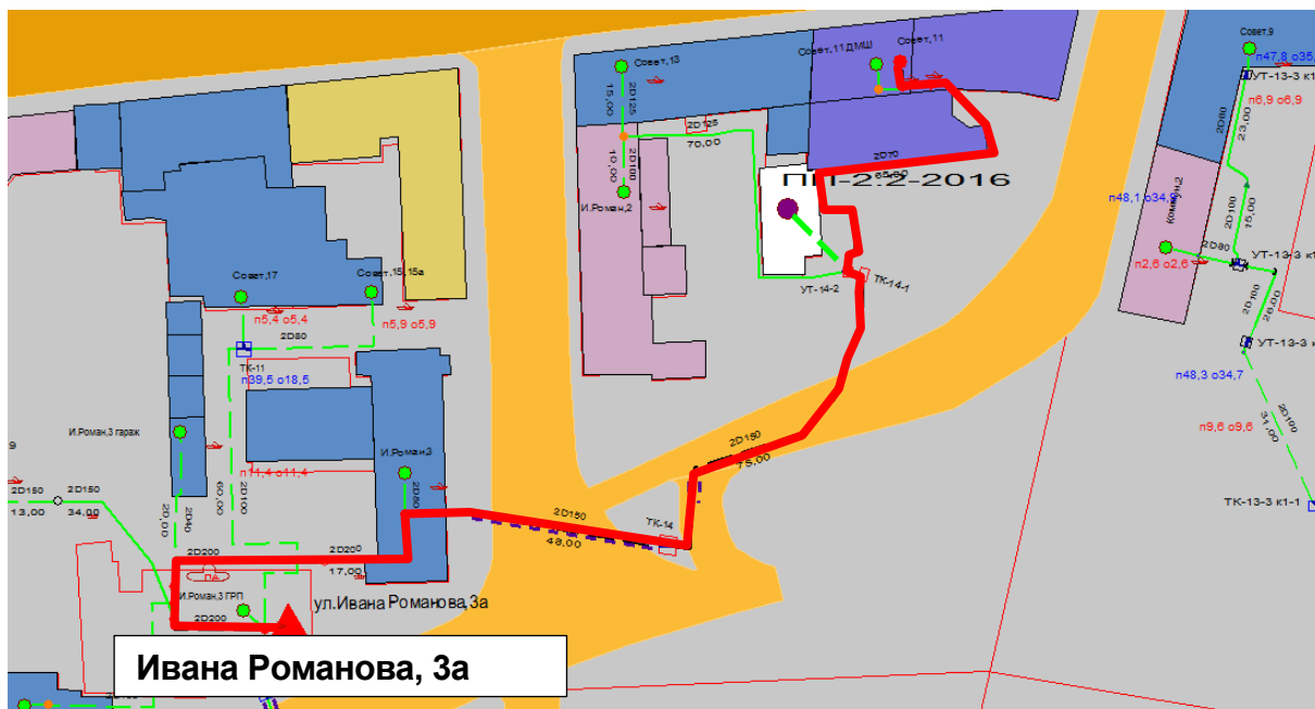
Рисунок 1.143 - Результат гидравлического расчета - расчетный путь теплоносителя от котельной Ивана Романова до ПТ-Совет, 11
