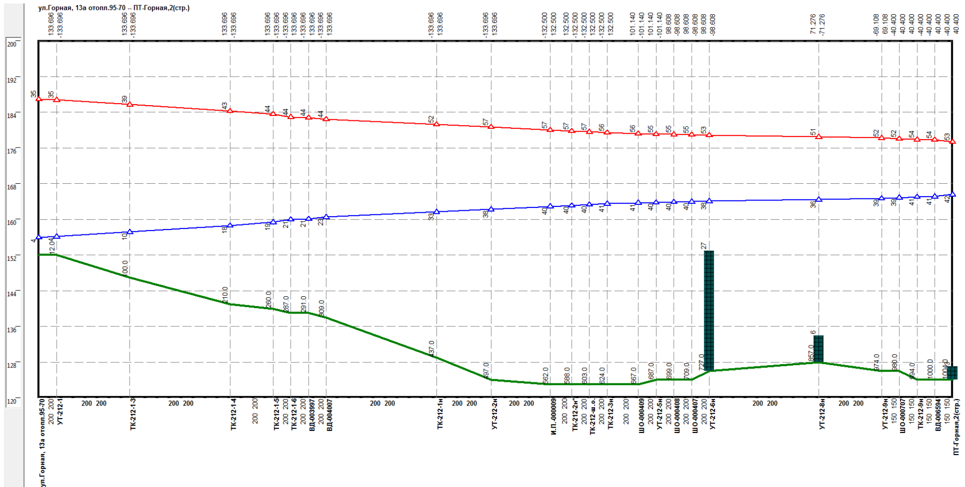
Рисунок Ошибка! Текст указанного стиля в документе отсутствует..178 –Результат гидравлического расчета - график гидравлических режимов по пути теплоносителя от котельной Горная, 13-а до ПТ-Горная,2(стр.)
