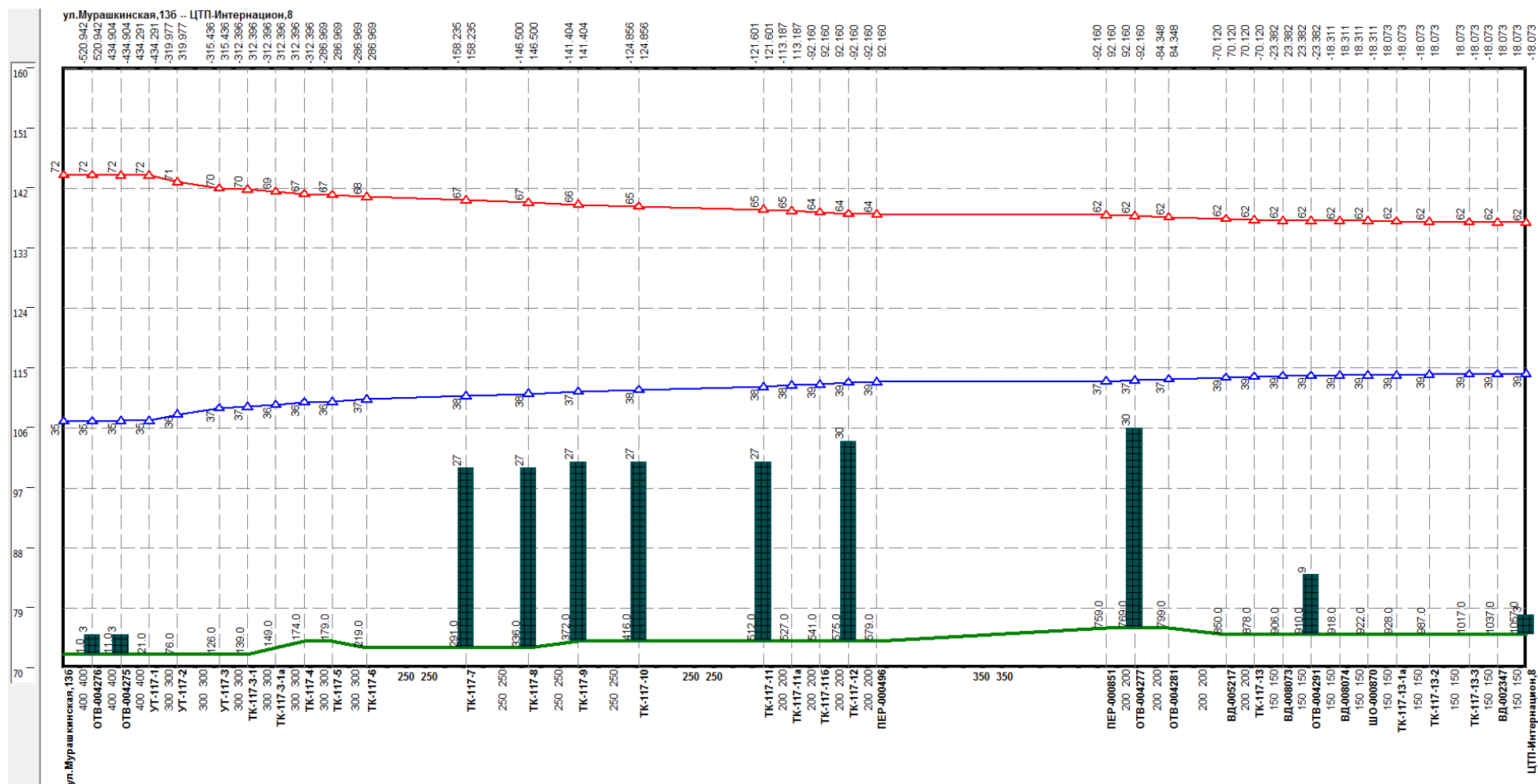
Рисунок Ошибка! Текст указанного стиля в документе отсутствует..154 –Результат гидравлического расчета - график гидравлических режимов по пути теплоносителя от котельной Мурашкинская, 13-б до ЦТП-Интернацион,8
