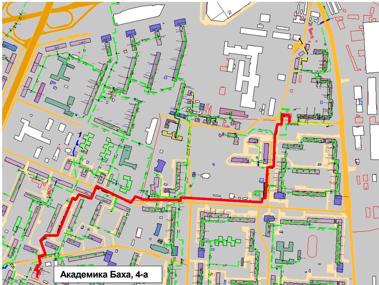
Рисунок Ошибка! Текст указанного стиля в документе отсутствует..205 – Результат гидравлического расчета - расчетный путь теплоносителя от котельной Академика Баха, 4-а до ПТ-ПП-1.84-2015
