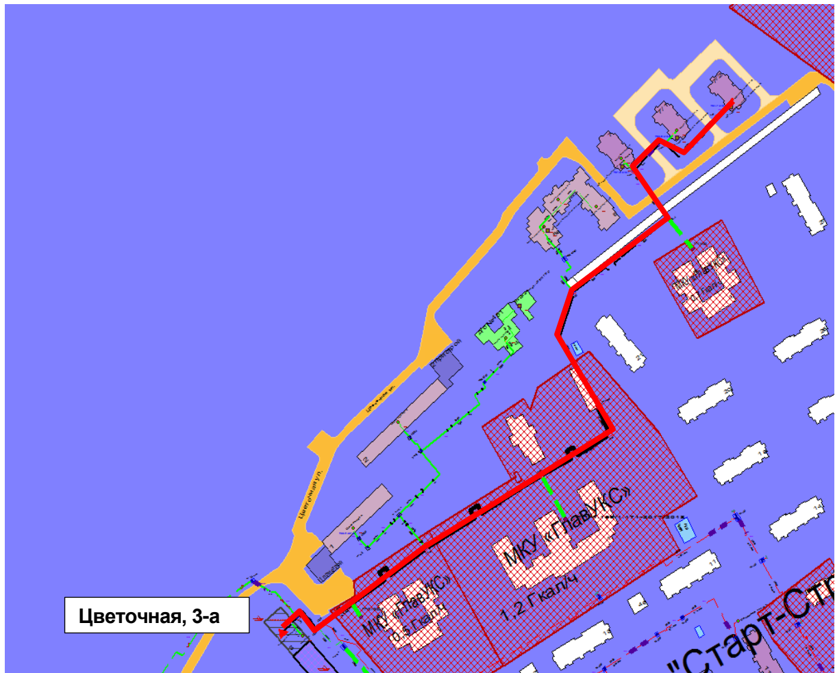
Рисунок Ошибка! Текст указанного стиля в документе отсутствует..221 – Результат гидравлического расчета - расчетный путь теплоносителя от котельной Цветочная, 3-а до ПТ-Цветочная,7/2
