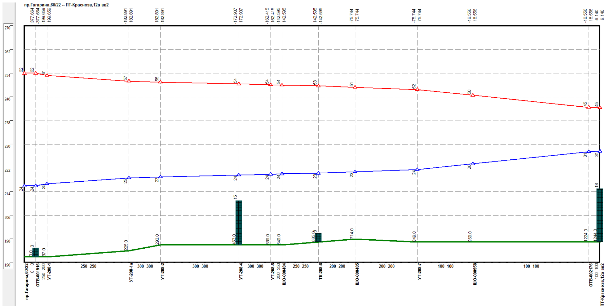
Рисунок Ошибка! Текст указанного стиля в документе отсутствует..172 –Результат гидравлического расчета - график гидравлических режимов по пути теплоносителя от котельной Гагарина, 60 к.22 до ПТ-Краснозв, 12а вв2
