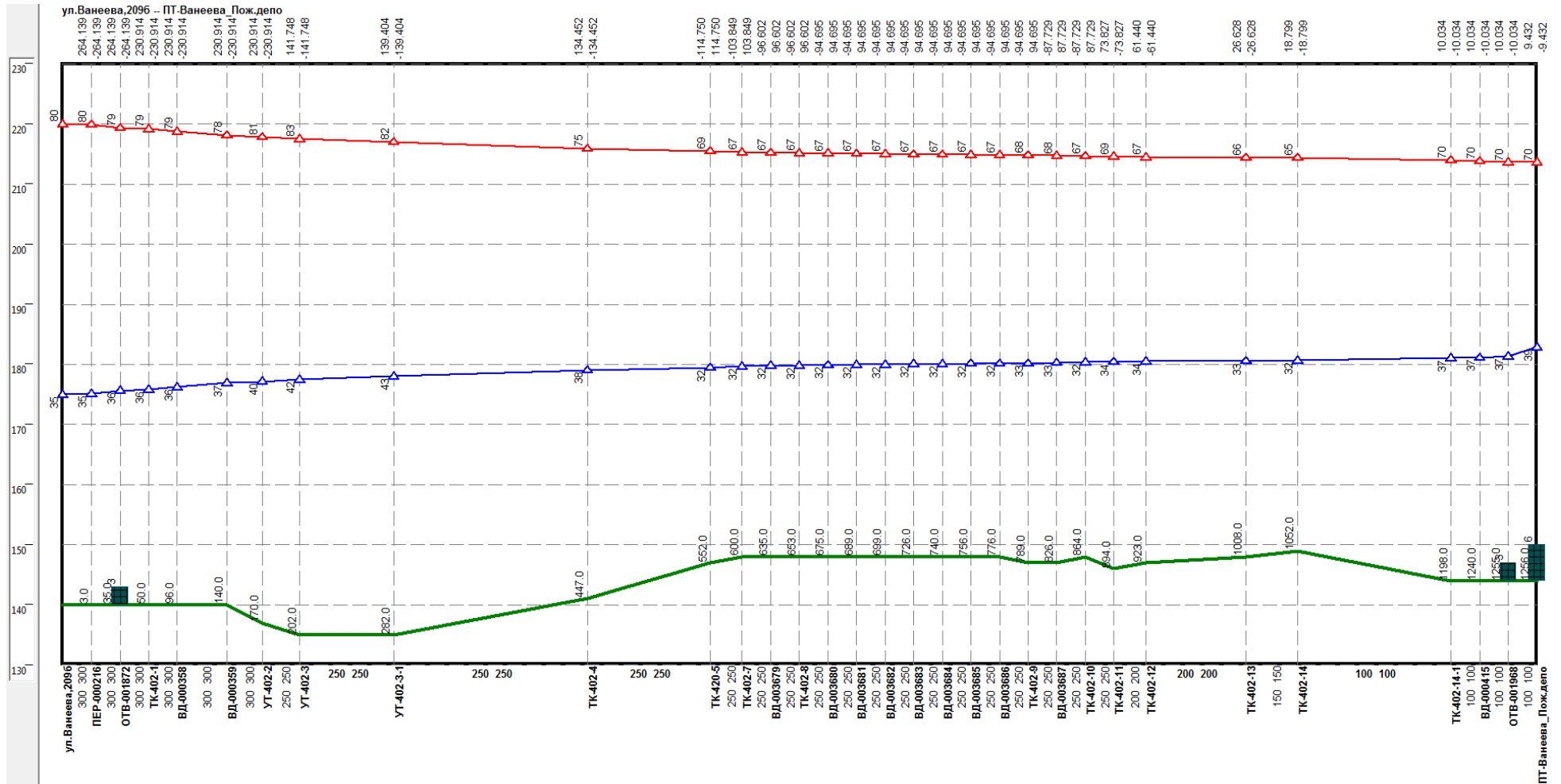
Рисунок Ошибка! Текст указанного стиля в документе отсутствует..176 –Результат гидравлического расчета - график гидравлических режимов по пути теплоносителя от котельной Ванеева, д.209-б до ПТ-Ванеева_Пож.депо
