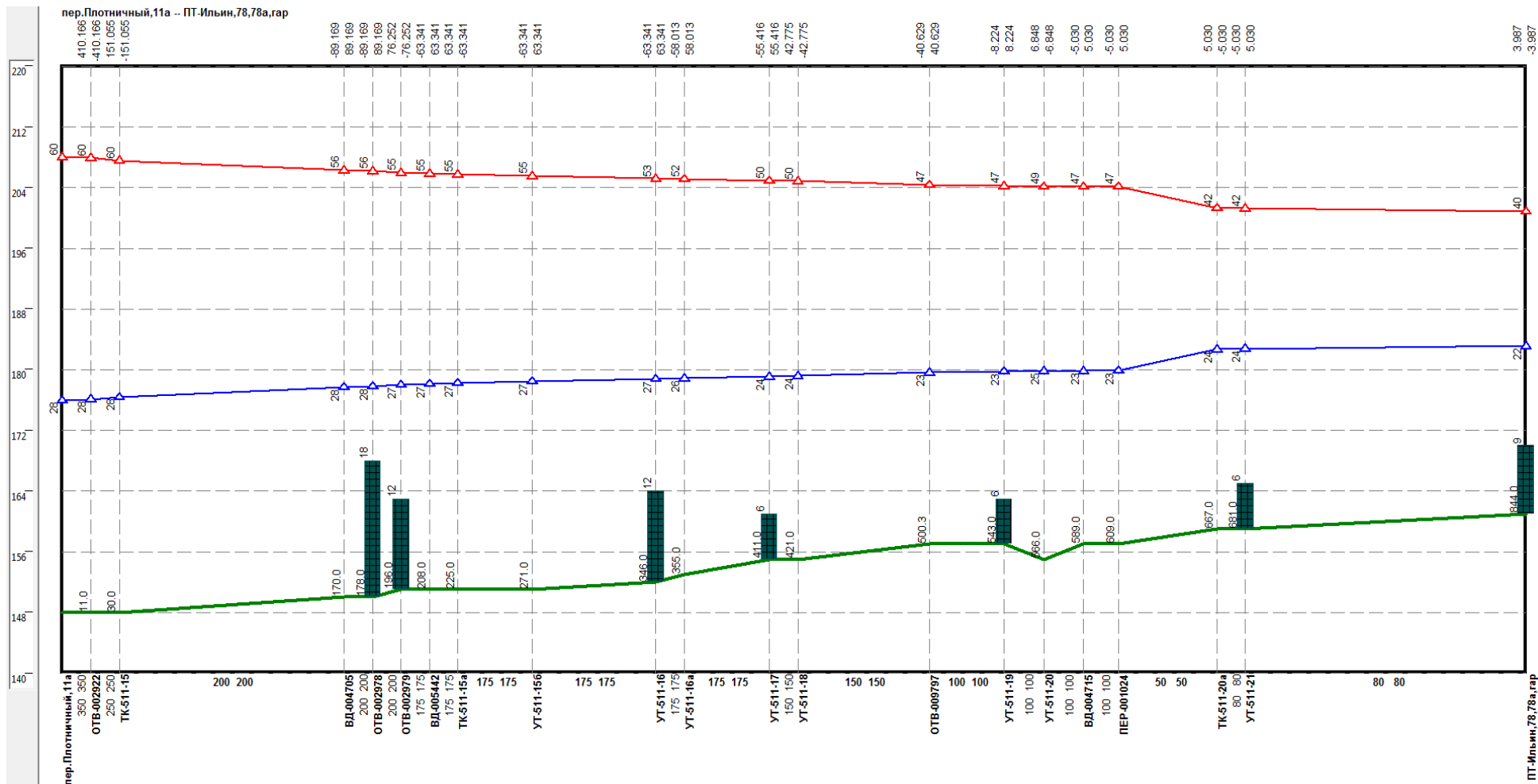
Рисунок Ошибка! Текст указанного стиля в документе отсутствует..182 –Результат гидравлического расчета - график гидравлических режимов по пути теплоносителя от котельной пер. Плотничный, 11 до ПТ-Ильин,78,78а,гар
